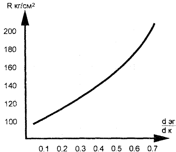
Рис. 2 Тарировочная зависимость отношения размера отпечатка на эталоне к размеру отпечатка на поверхности конструкции от прочности бетона
