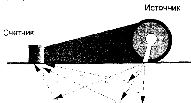
Рис. 5. Схема поверхностного просвечивания (рассеяния)
