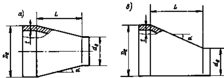
Черт. 2. Переходы
