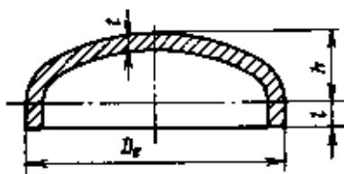
Черт. 6. Эллиптическая заглушка
