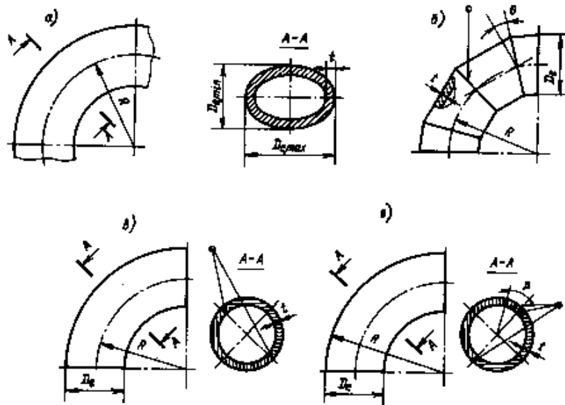
Черт.1. Отводы
