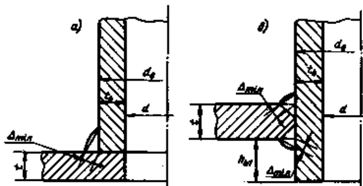
Черт. 4. Типы сварных соединений тройников со штуцером
