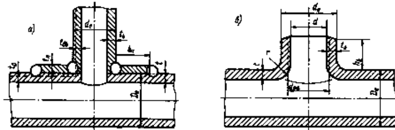
Черт. 3. Тройники
