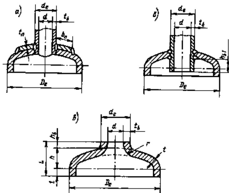
Черт. 7. Эллиптические заглушки со штуцером а - с укрепляющей накладкой; б - пропущенным внутрь заглушки; в - с отбортованным отверстием
