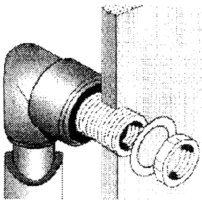
Переходный угольник (наружная/ внутренняя резьба) для пустотелых стен с длиной резьбы 30 мм.
