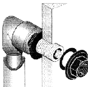
Деталь для подключения на пустотелых стенах с переходным угольником.
