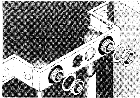
Двойной монтажный узел, включая 2 переходных угольника (наружная/ внутренняя резьба) с контргайкой, уплотнением и прижимной шайбой.
