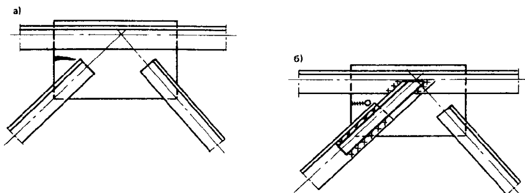
Рис. 27. Установка «энергетического мостика» для предотвращения распространения трещины
