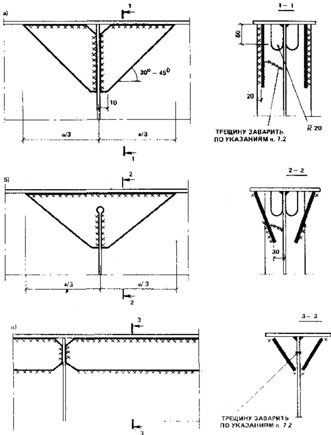
Рис. 30. Усиление верхней зоны подкрановых балок a-в - варианты усиления
