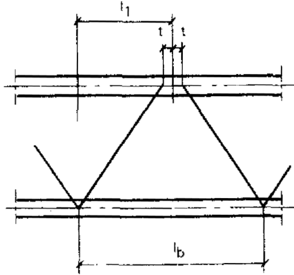
Рис. 2. Сквозной стержень с расцентровкой решетки
