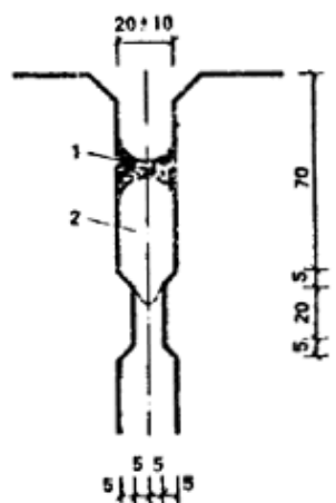
Рис. 29. Схема герметизации устья вертикального закрытого стыка при применении отверждающих герметизирующих мастик
