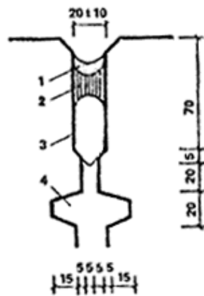
Рис. 33. Схема герметизации устья вертикального дренажного стыка
