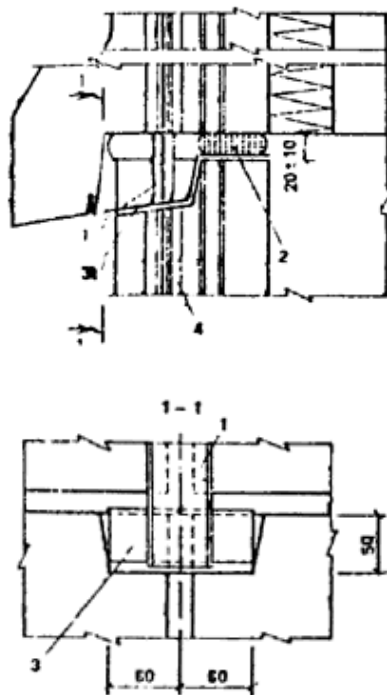
Рис. 39. Схема герметизации устья горизонтального открытого стыка с выносным противодождовым зубом
