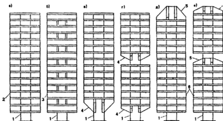
Рис. 5. Ствольные конструктивные системы (с одним несущим стволом)
