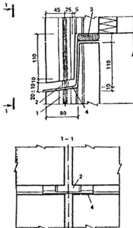
Рис. 37. Схемы изоляции устья вертикального открытого стыка резиновым профилем a — без смещения плоскостей сопрягаемых панелей; б — при допустимом смещении плоскостей сопрягаемых панелей 1 — резиновый профиль
