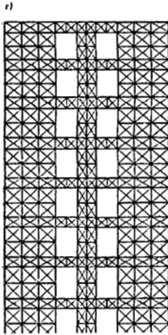
Рис. 22. Двухмерные (плоские) расчетные схемы бескаркасных зданий
