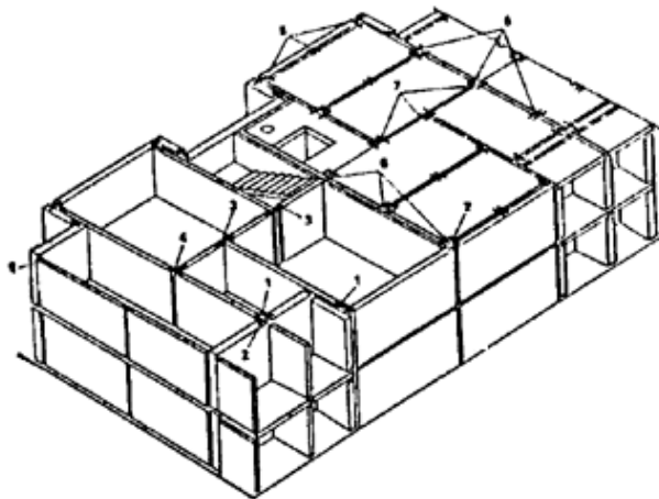
Рис. 6. Схема расположения связей в крупнопанельном здании
