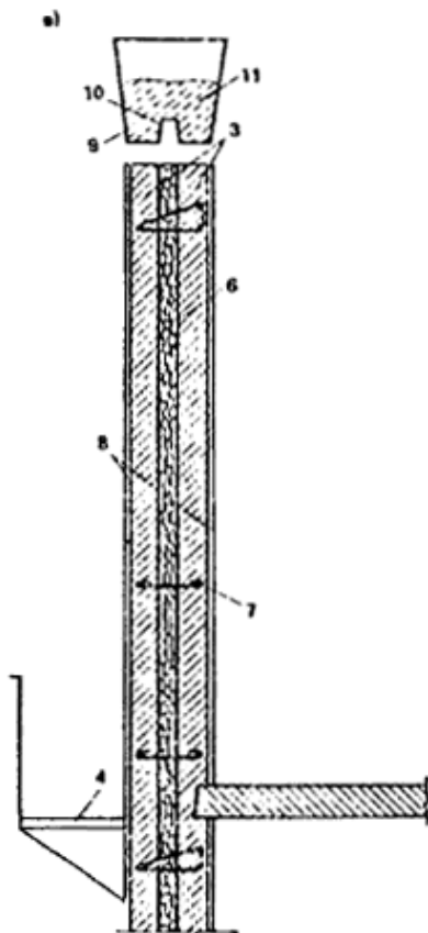
Рис. 26. Наружные стены монолитных зданий
