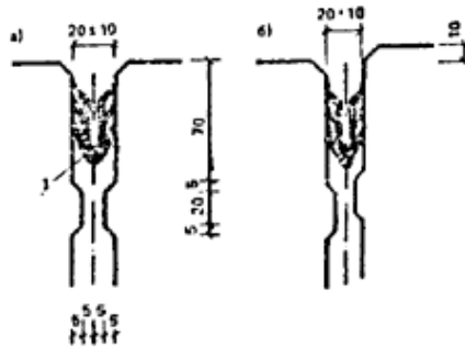
Рис. 37. Схемы изоляции устья вертикального открытого стыка резиновым профилем a — без смещения плоскостей сопрягаемых панелей; б — при допустимом смещении плоскостей сопрягаемых панелей 1 — резиновый профиль
