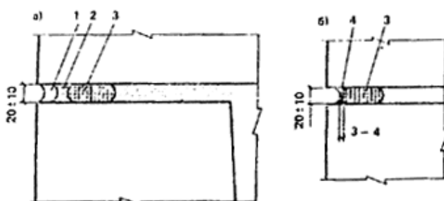
Рис. 31. Схема герметизации устья плоского горизонтального закрытого стыка
