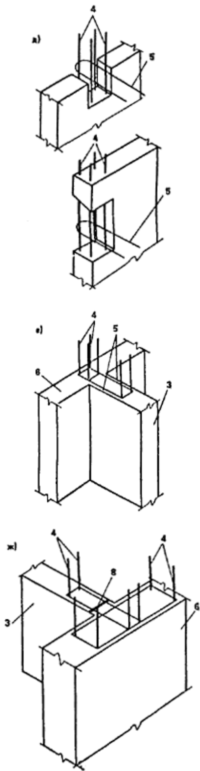
Рис. 15. Вертикальные торцевые (а — в), фронтальные (г — е) и фронтально-торцевые (ж) узлы
