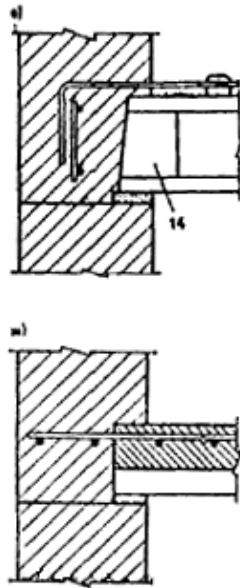
Рис. 20. Комбинированные узлы наружных монолитных стен со сборными многопустотными и сборно-монолитными перекрытиями
