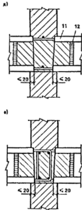
Рис. 16. Контактные узлы внутренних монолитных стен
