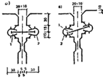
Рис. 36. Схемы изоляции устья вертикального открытого стыка с применением жесткого водоотбойного экрана a — без смещения плоскостей сопрягаемых панелей; б — при допустимом смещении плоскостей сопрягаемых панелей 1 — жесткий водоотбойный экран из пластмасс на основе ПВХ; 2 — направляющий профиль из того же материала
