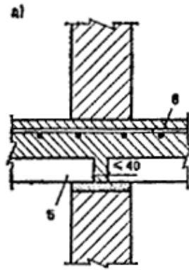
Рис. 18. Платформенные узлы внутренних монолитных стен
