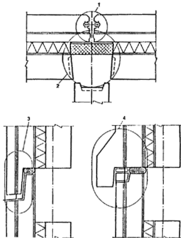
Рис. 35. Открытый стык наружных стеновых панелей 1 — узел (см. рис. 36, 37); 2 — узел (см. рис. 40); 3 — узел (см. рис. 33); 4 — узел (см. рис. 39)
