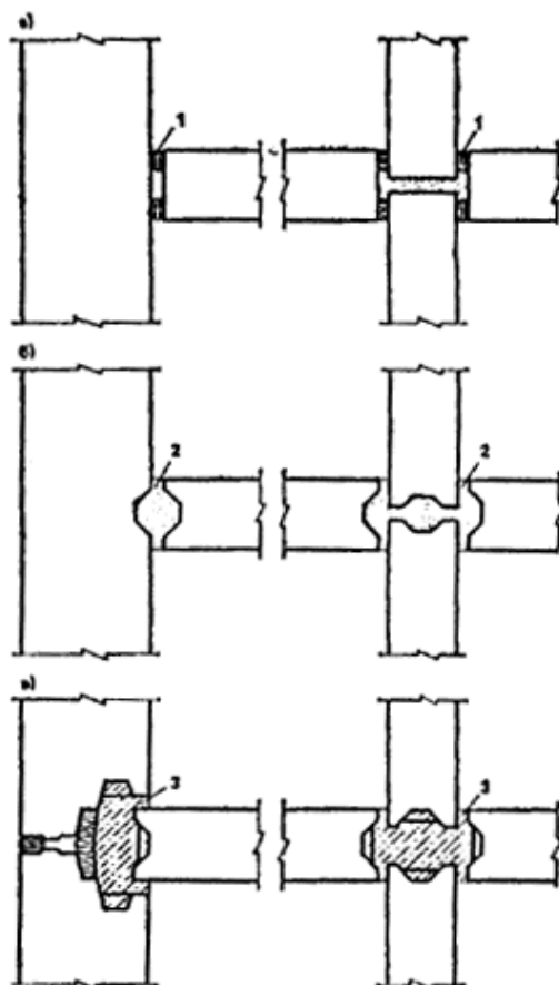
Рис. 12. Типы вертикальных стыков панельных стен
