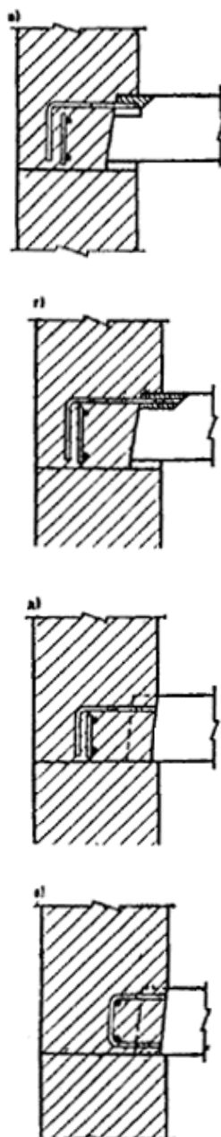
Рис. 21. Комбинированные узлы монолитных стен со сборными сплошными плитами перекрытий
