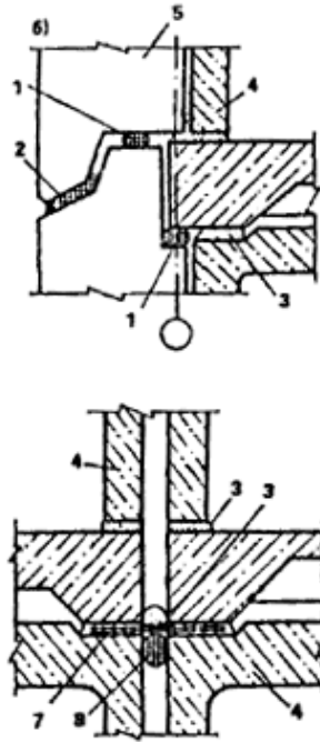
Рис. 13. Горизонтальные стыки объемно-блочных зданий
