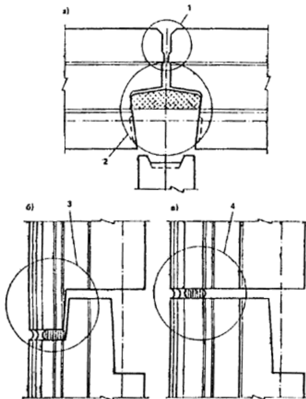
Рис. 27. Закрытый стык наружных стеновых панелей
