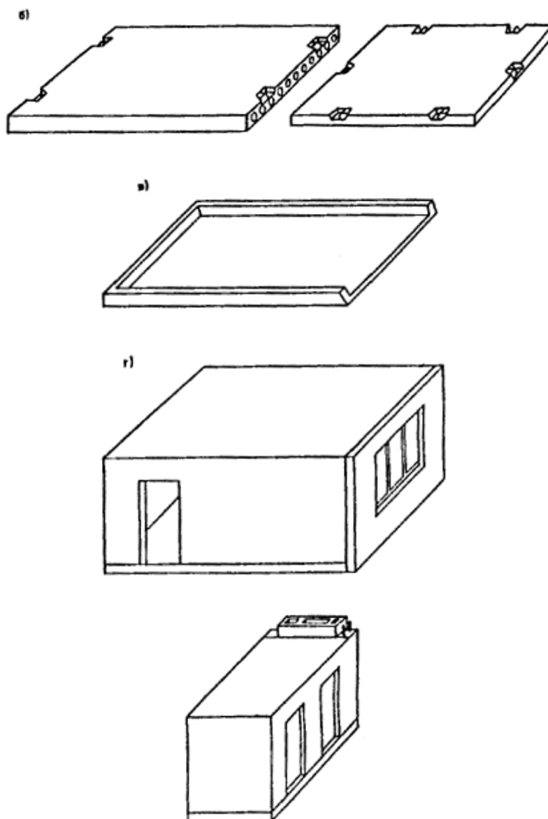
Рис. 1. Крупноразмерные сборные элементы жилых зданий
