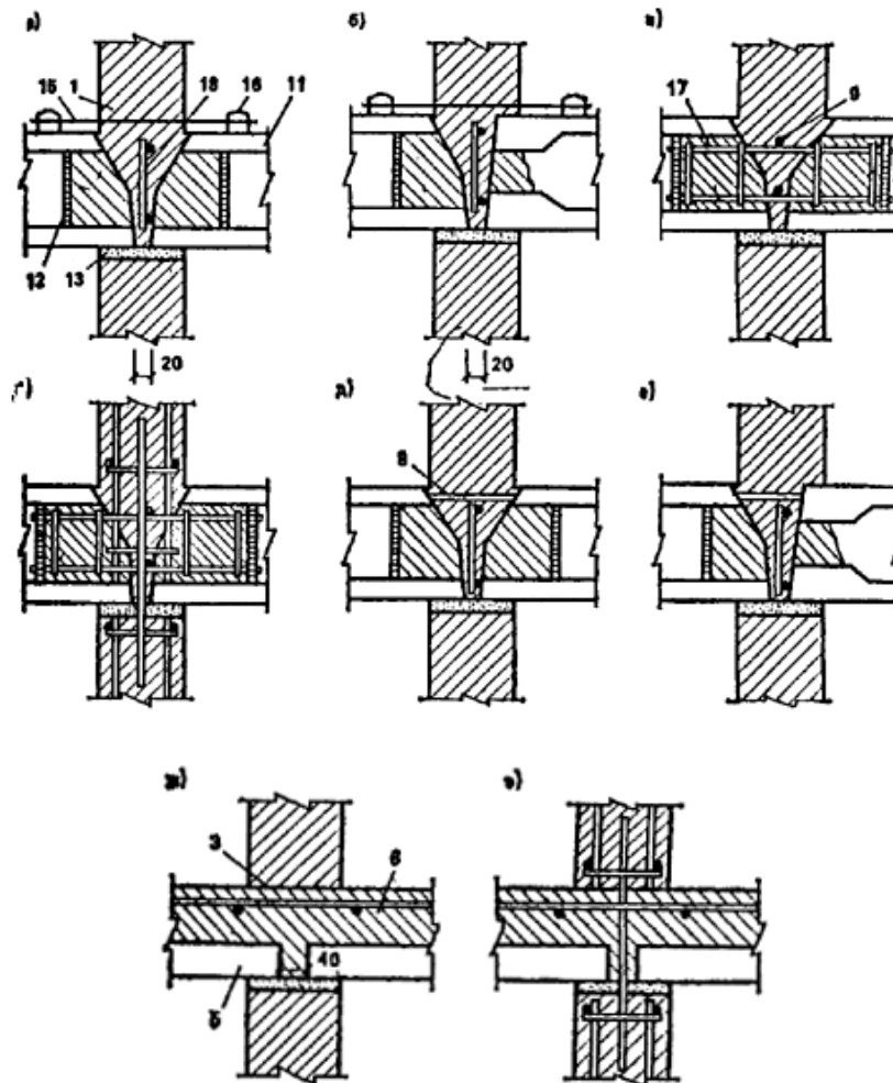
Рис. 19. Комбинированные узлы внутренних монолитных стен
