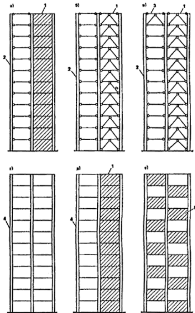
Рис. 4. Каркасные конструктивные системы
