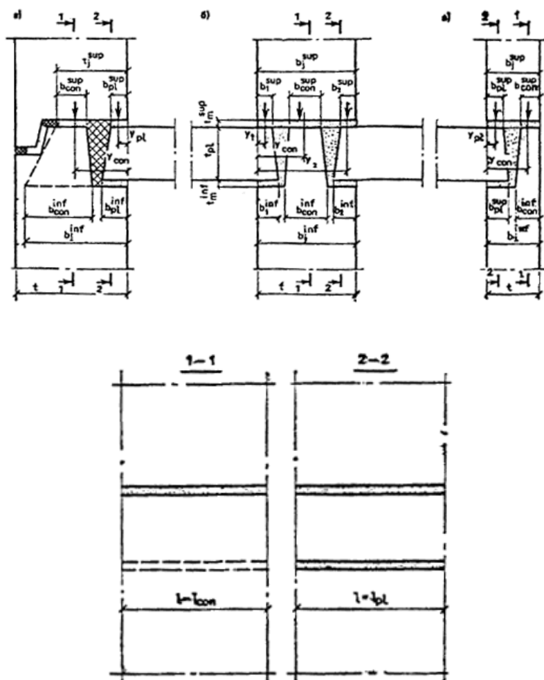
Рис. 10. Контактно-платформенные стыки сборных стен
