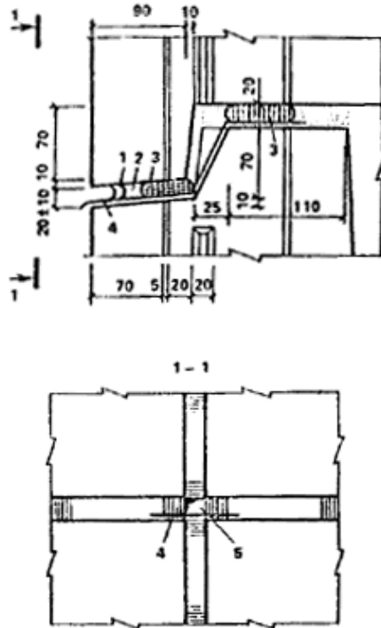
Рис. 34. Схема герметизации устья горизонтального дренированного стыка 1 — защитное покрытие; 2 — нетвердеющая герметизирующая мастика; 3 — уплотняющая прокладка при зазоре стыка 20 мм — 30 — 40 мм, при зазоре 10 мм — 20 мм, при зазоре 30 мм — 40 — 50 мм; 4 — водоотводящий фартук; 5 — дренажное отверстие
