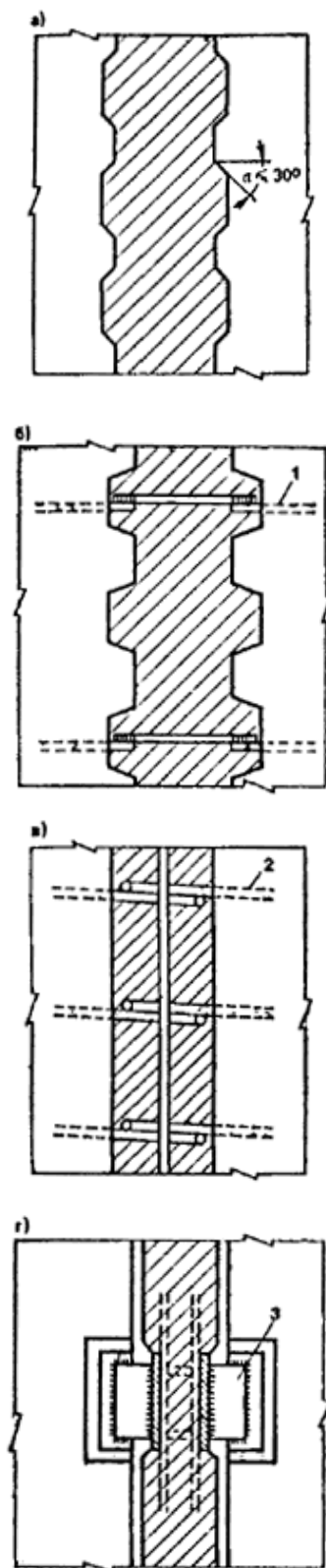
Рис. 11. Схемы восприятия сдвигающих усилий в вертикальном стыке панельных стен
