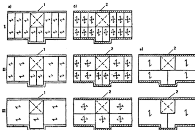
Рис. 3. Стеновые конструктивные системы
