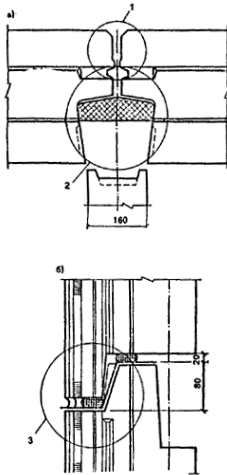
Рис. 32. Дренажный стык наружных стеновых панелей
