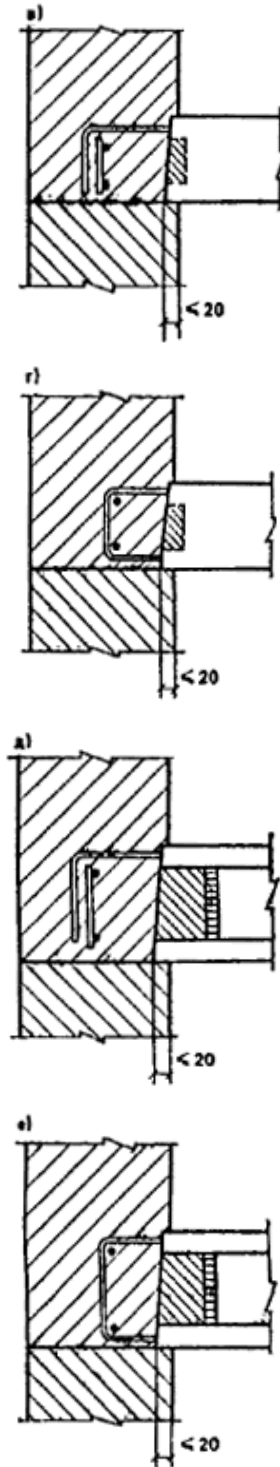
Рис. 17. Контактные узлы наружных монолитных стен
