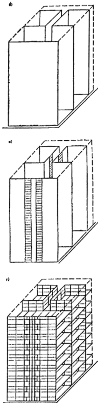
Рис. 23. Пространственные (трехмерные) расчетные схемы бескаркасных зданий.
