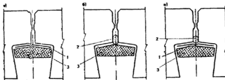
Рис. 40. Варианты устройства воздухозащитной изоляции с применением a — воздухозащитной ленты; б — уплотняющей прокладки; в — комбинированной 1 — воздухозащитная лента; 2 — уплотняющая прокладка на клее типа КН; 3 — теплоизоляция
