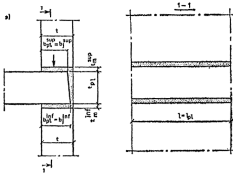
Рис. 7 Платформенные стыки сборных стен
