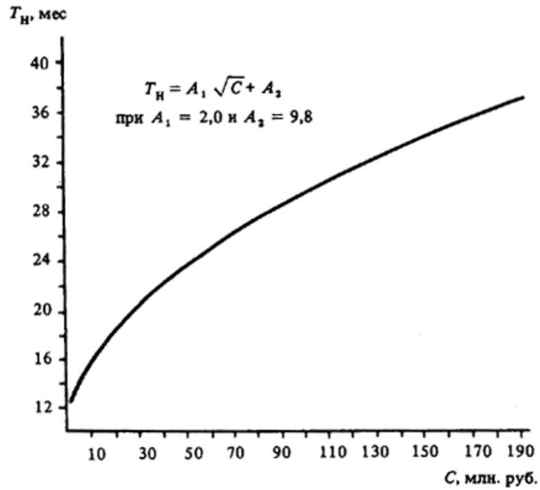
Черт. 11. Определение T_n объектов по отрасли в целом при C = 2 - 190 млн. руб.
