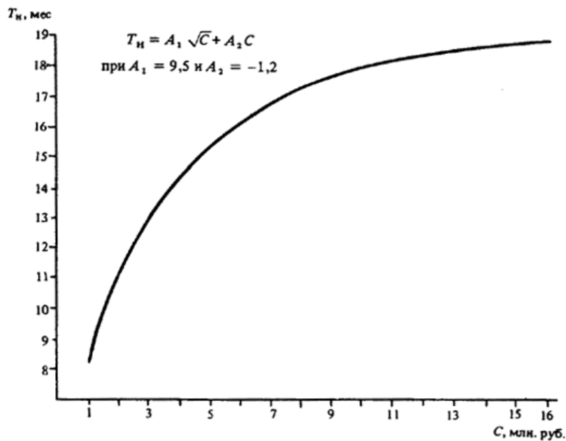
Черт. 56. Определение T_n различных объектов при C = 1 - 16 млн. руб.
