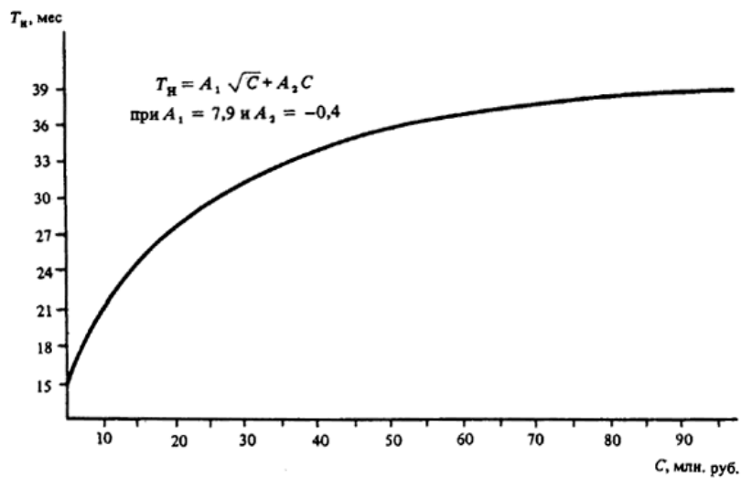
Черт. 16. Определение T_n различных объектов
