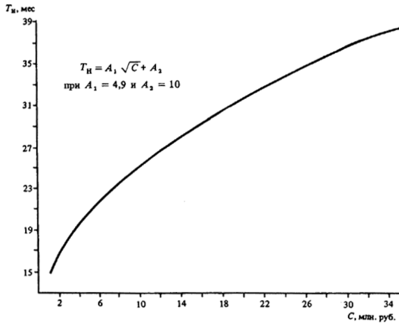
Черт. 32. Определение T_n различных объектов при C = 1 - 36 млн. руб.
