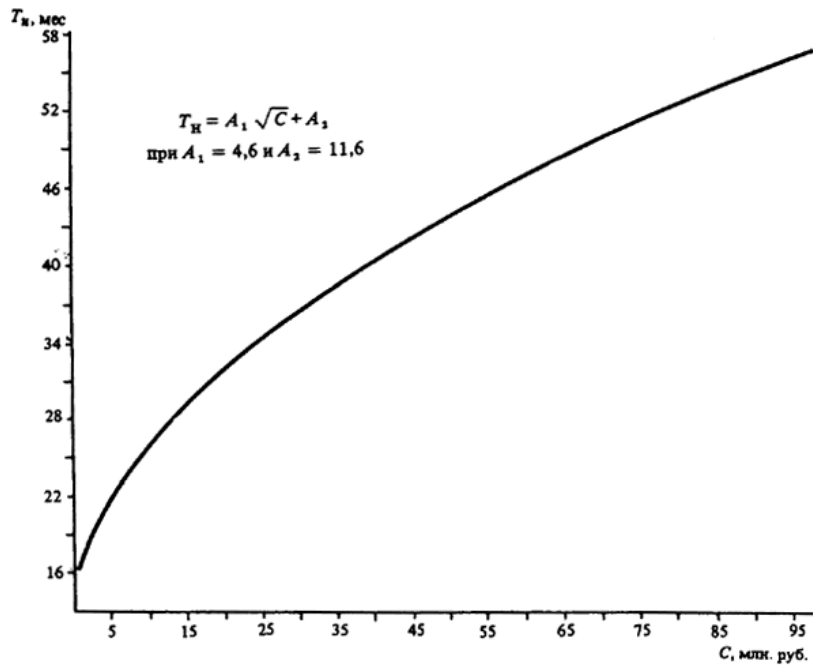
Черт. 28. Определение T_n различных объектов при C = 1 - 100 млн. руб.
