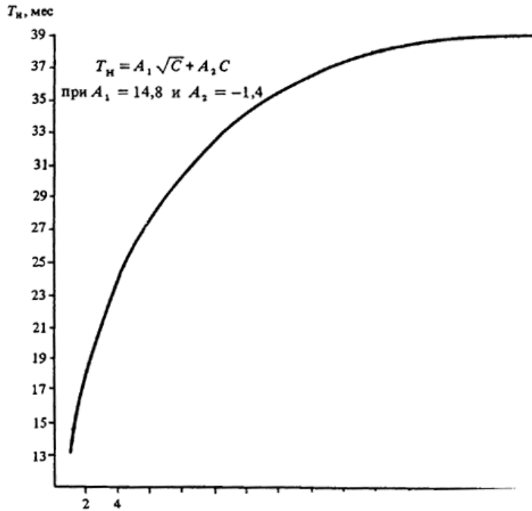
Черт. 33. Определение T_n различных объектов при C = 1 - 30 млн. руб.
