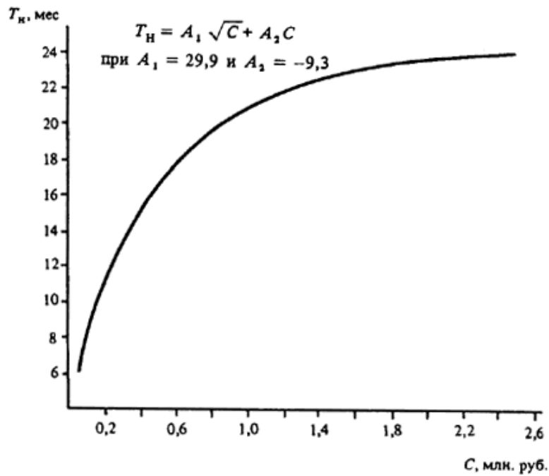
Черт. 58. Определение T_n объектов общественного питания и рынков при C = 0,05 - 2,40 млн. руб.
