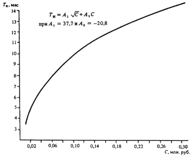
Черт. 52. Определение T_n различных объектов при C = 0,01 - 0,30 млн. руб.
