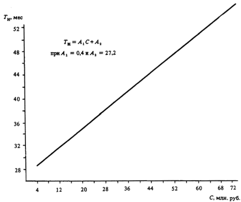
Черт. 19. Определение T_n различных объектов при C = 4 - 72 млн. руб.
