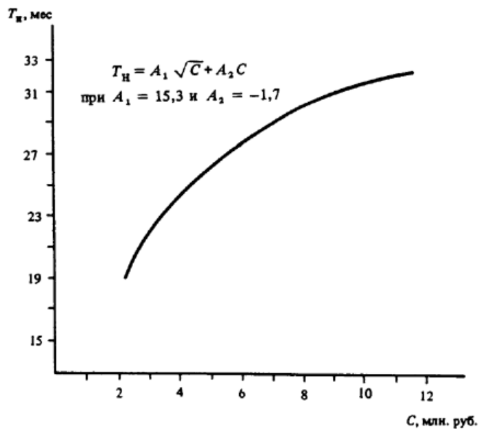
Черт. 4. Определение T_n электроподстанций при C = 1,1 - 12,0 млн. руб.
