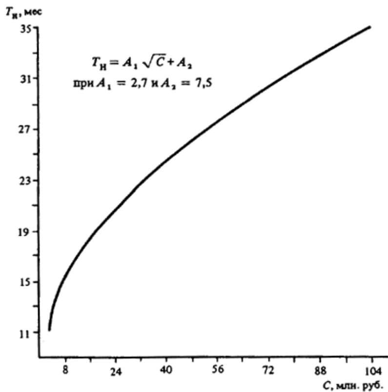
Черт. 25. Определение T_n различных объектов при C = 2 - 104 млн. руб.
