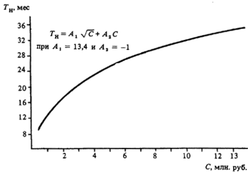
Черт. 50. Определение T_n различных объектов при C = 0,5-13,0 млн. руб.
