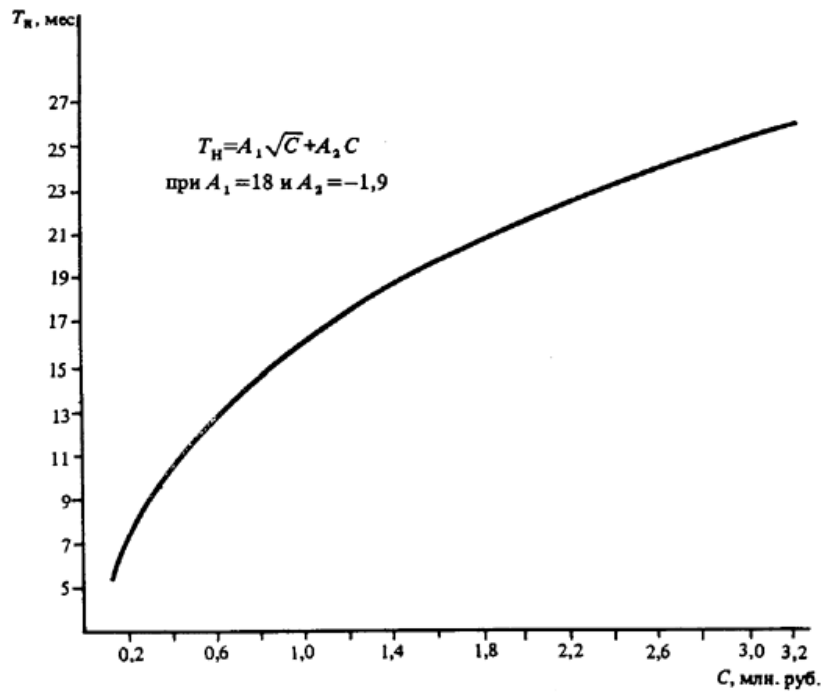
Черт. 49. Определение T_n предприятий материально-технического обеспечения при C = 0,1 - 3,2 млн. руб.
