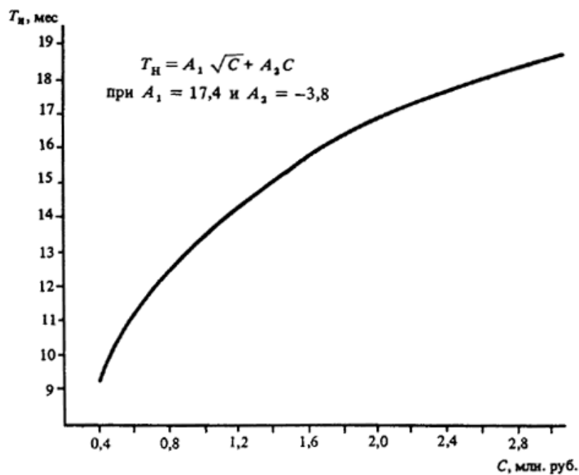
Черт. 41. Определение T_n различных объектов при C = 0,4 - 3,0 млн. руб.
