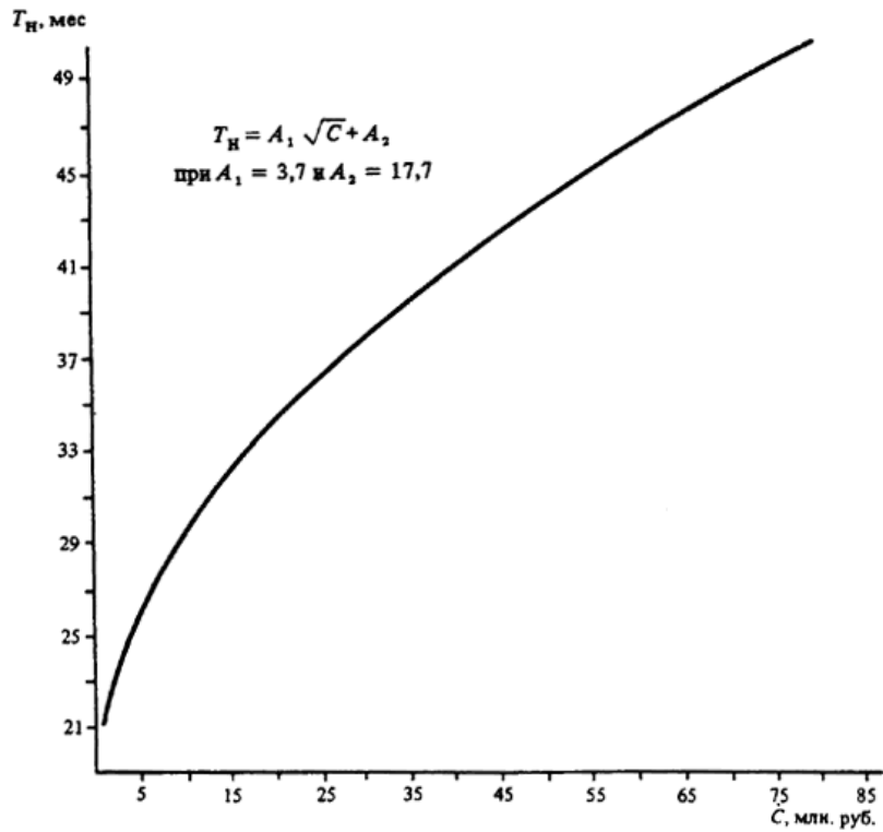
Черт. 15. Определение T_n различных объектов при C = 1 - 80 млн. руб.
