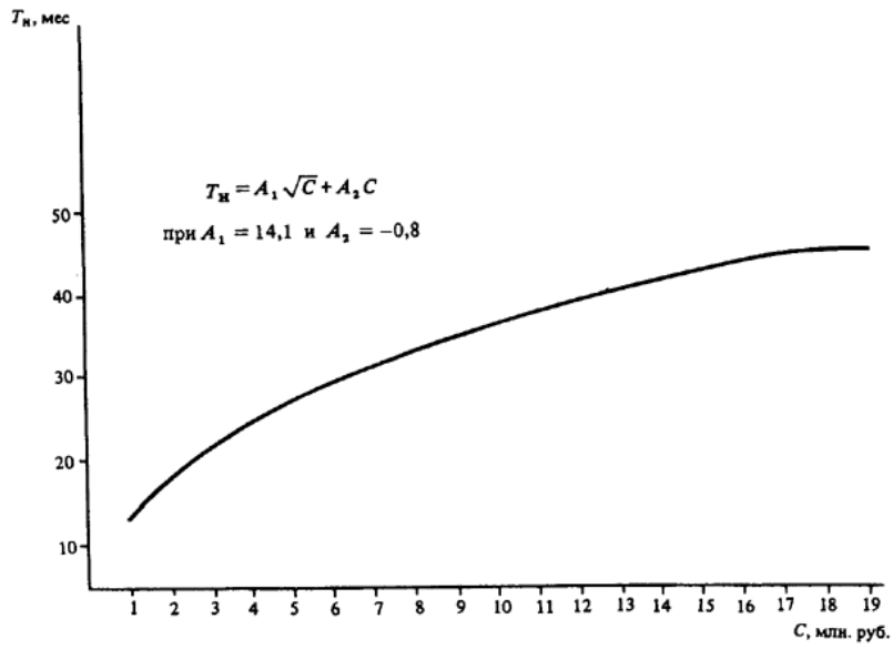
Черт. 34. Определение T_n различных объектов при C = 1 - 19 млн. руб.
