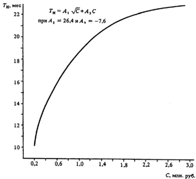
Черт. 59. Определение T_n объектов розничной торговли и непродовольственных магазинов при C = 0,2 - 2,8 млн. руб.
