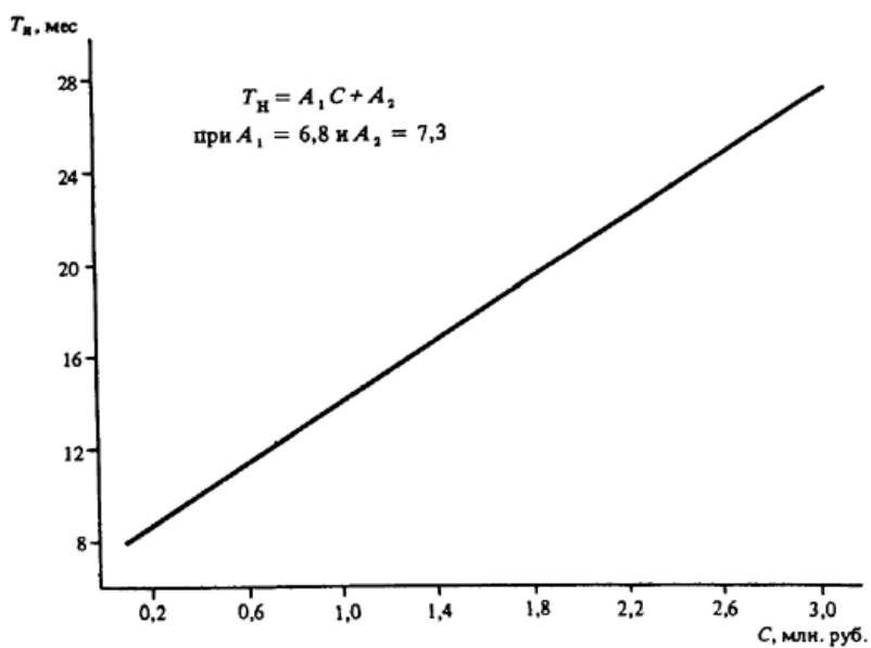
Черт. 48. Определение T_n предприятий по ремонту и обслуживанию сельхозтехники при C = 0,1 - 3,0 млн. руб.
