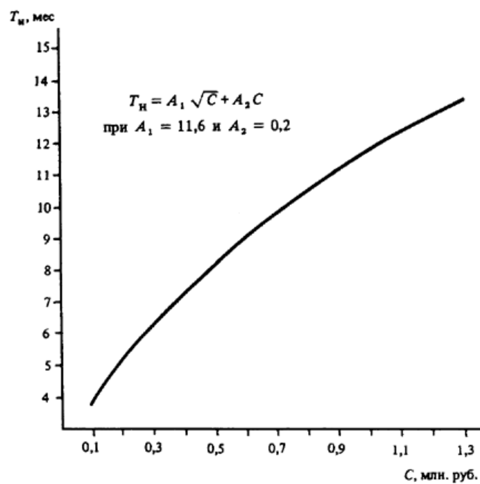
Черт. 3. Определение T_n электроподстанций при C = 0,1 - 1,3 млн. руб.
