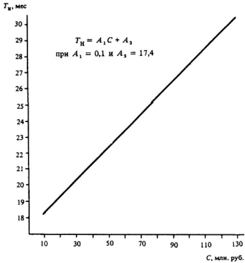
Черт. 10. Определение T_H объектов проката готовой продукции при C = 10 - 130 млн. руб.
