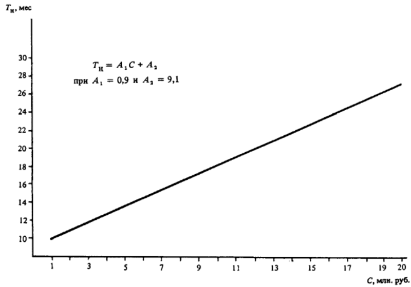
Черт. 2. Определение T_n ТЭС при C = 1 - 20 млн. руб.
