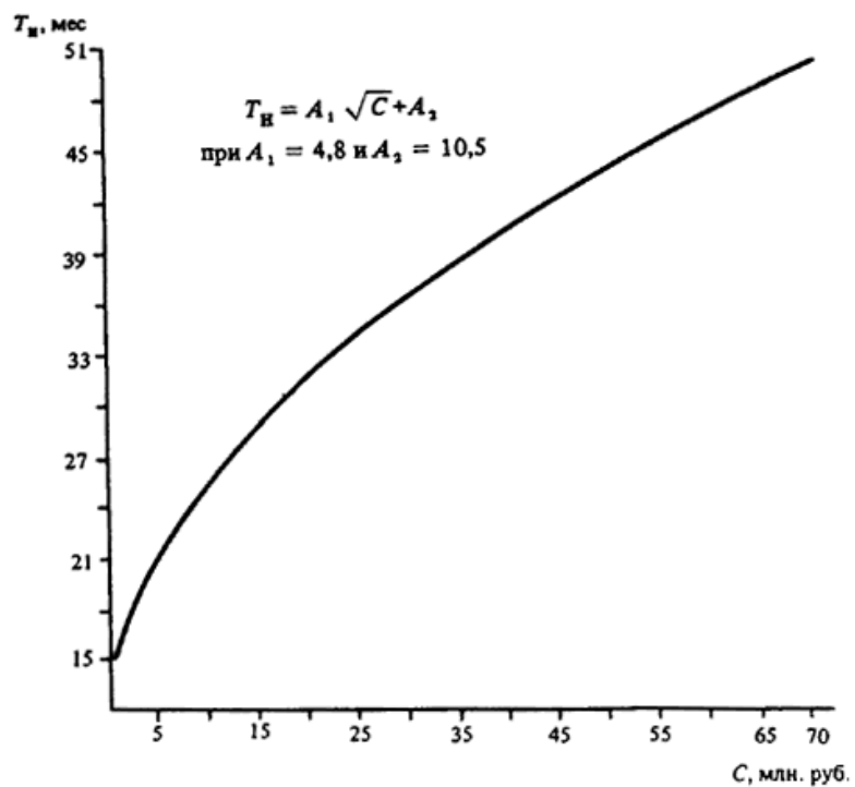
Черт. 13. Определение T_n различных объектов при C = 1 - 70 млн. руб.
