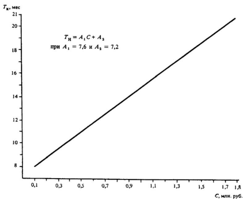
Черт. 6. Определение T_n баз производственного обслуживания при C = 0,1 - 1,8 млн. руб.
