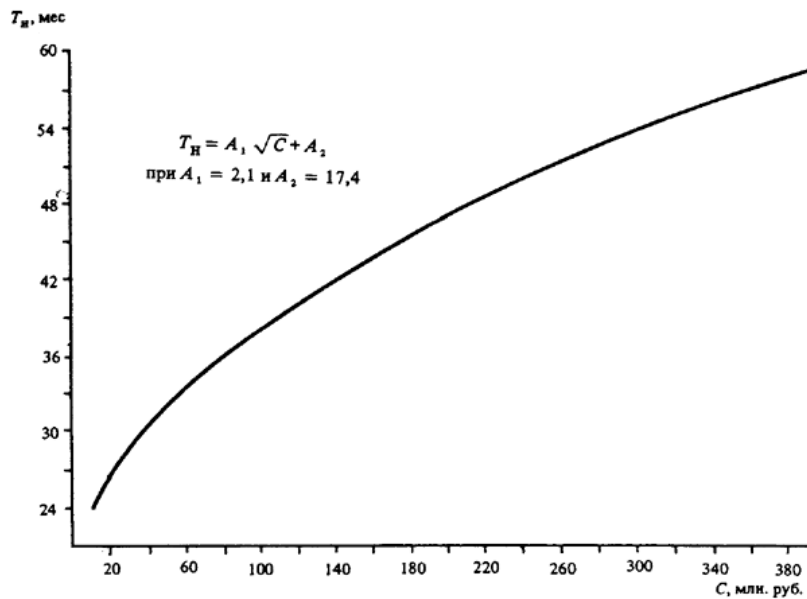
Черт. 24. Определение T_n различных объектов при C = 10 - 400 млн. руб.
