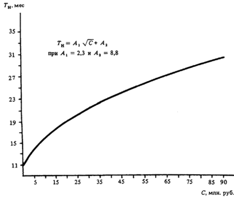
Черт. 9. Определение T_n сталеплавильного, ферросплавного и огнеупорного производства при C = 1 - 90 млн. руб.
