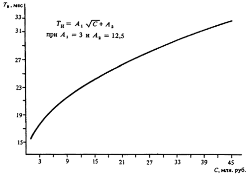
Черт. 55. Определение T_n объектов воздушного транспорта при C = 1 - 45 млн. руб.
