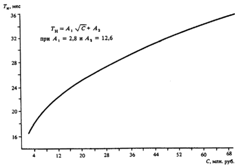
Черт. 12. Определение T_n различных объектов при C = 2 - 72 млн. руб.
