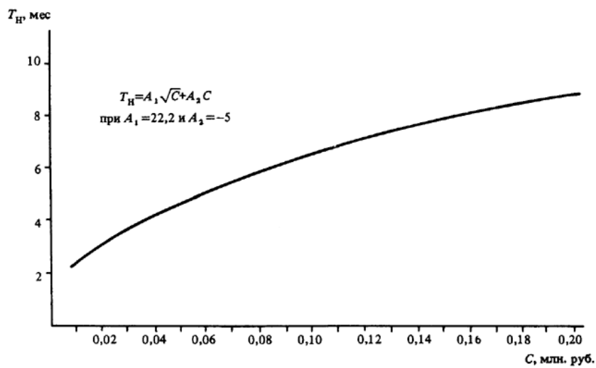
Черт. 47. Определение T_n прочих объектов
