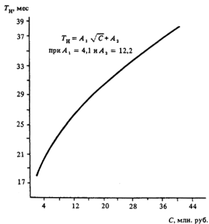
Черт. 17. Определение T_n различных объектов при C = 2 - 40 млн. руб.
