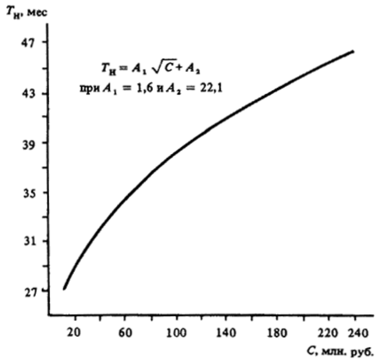
Черт. 23. Определение T_n различных объектов при C = 10 - 240 млн. руб.
