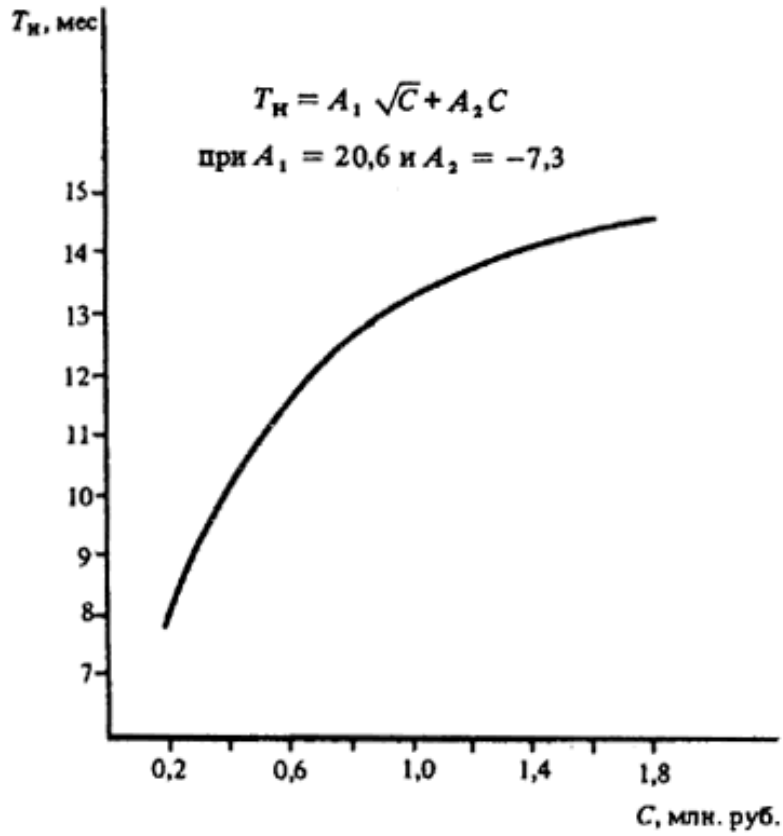
Черт. 54. Определение T_n объектов морского транспорта при C = 0,2 - 1,8 млн. руб.
