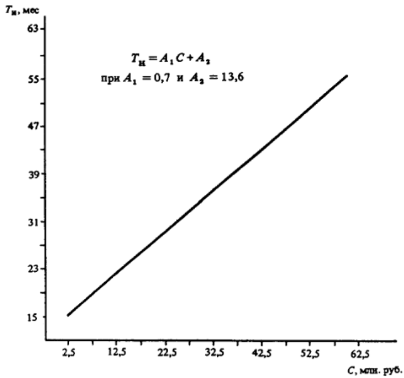
Черт. 39. Определение T_n различных объектов при C = 2,5 - 60,0 млн. руб.
