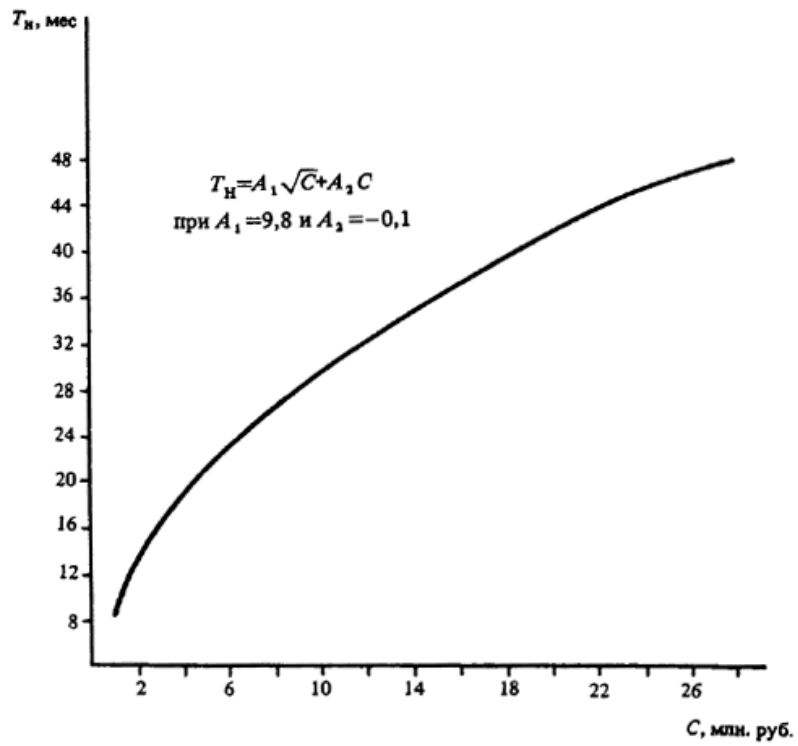
Черт. 45. Определение T_n птицеводческих ферм, птицефабрик при C = 1 - 27 млн. руб.
