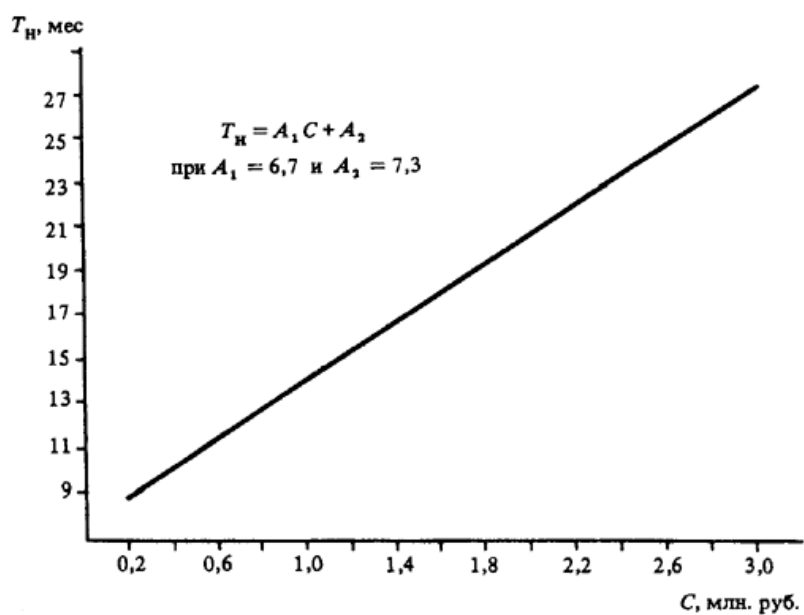
Черт. 40. Определение T_n различных объектов
