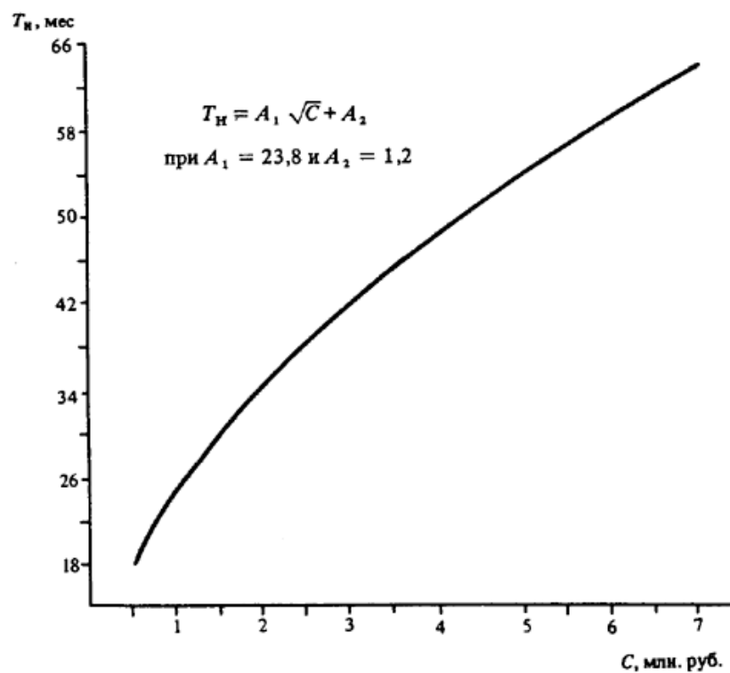
Черт. 57. Определение T_n различных объектов при C = 0,5 - 7,0 млн. руб.
