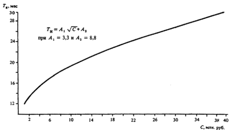
Черт. 7. Определение T_n различных объектов при C = 1 - 40 млн. руб.
