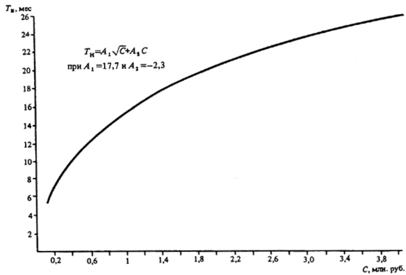
Черт. 44. Определение T_n объектов свиноводства при C = 0,1 - 4,0 млн. руб.
