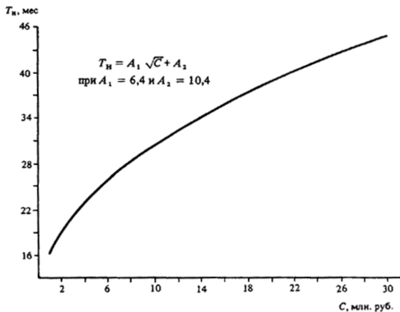
Черт. 31. Определение T_n различных объектов при C = 1 - 30 млн. руб.
