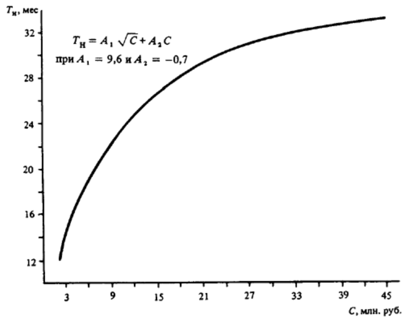
Черт. 14. Определение T_n различных объектов при C = 2 - 45 млн. руб.
