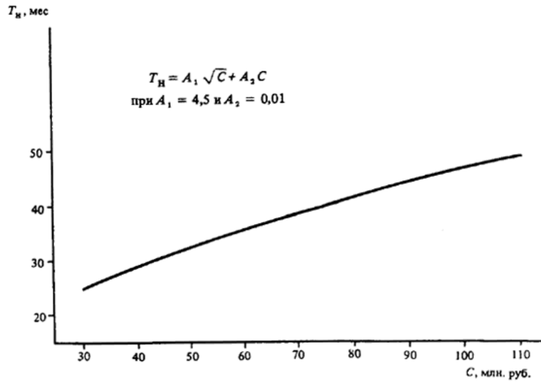
Черт. 1. Определение T_n ГРЭС при C = 30 - 110 млн. руб.
