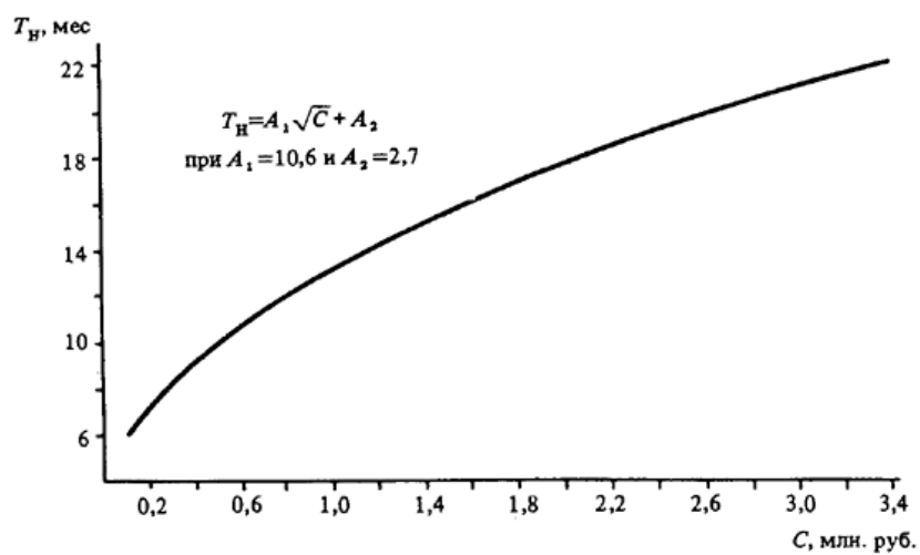
Черт. 42. Определение T_n объектов животноводства при C = 0,1-3,4 млн. руб.
