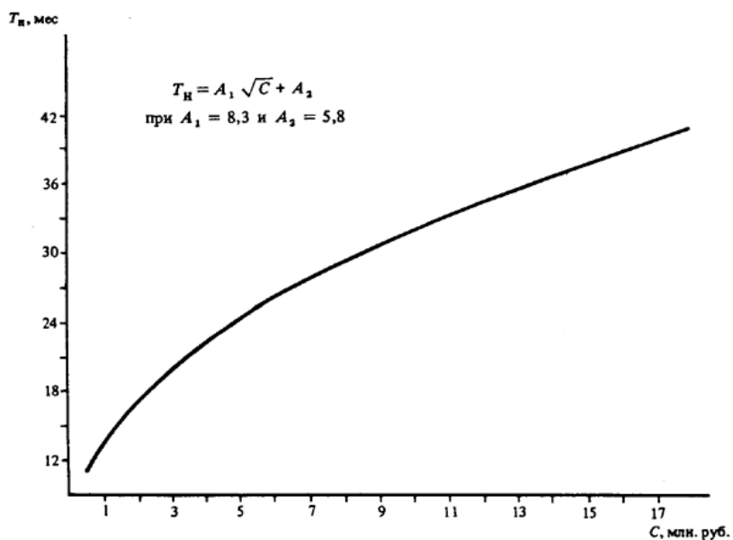
Черт. 51. Определение T_n предприятий по хранению и обработке картофеля, фруктов и овощей при C = 0,5 - 18,0 млн. руб.
