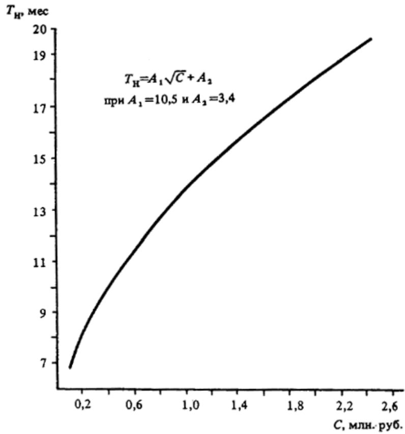
Черт. 43. Определение T_n овцеводческих ферм при C = 0,1 - 2,4 млн. руб.
