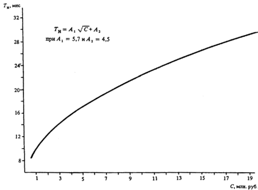
Черт. 26. Определение T_n различных объектов при C = 0,5 - 20,0 млн. руб.
