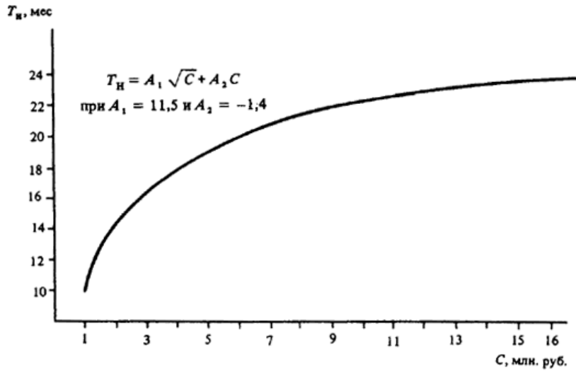
Черт. 22. Определение T_n отдельных цехов, корпусов и зданий при C = 1 - 16 млн. руб.
