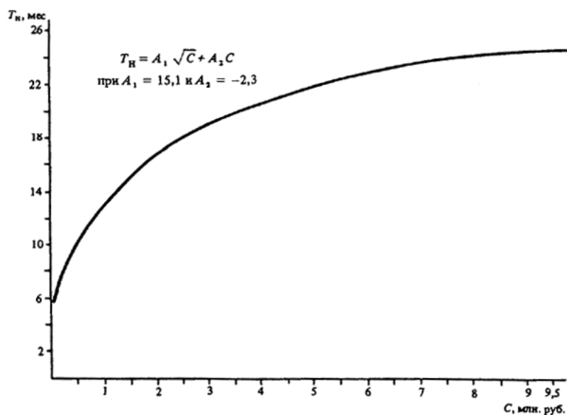
Черт. 30. Определение T_n различных объектов при C = 0,1 - 11,0 млн. руб.
