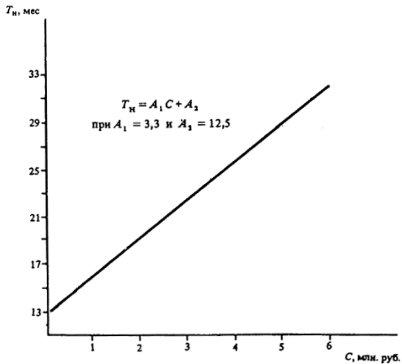
Черт. 36. Определение T_n различных объектов при C = 0,1 - 6,0 млн. руб.
