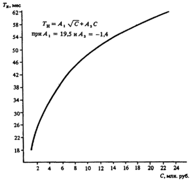
Черт. 27. Определение T_n лесозаготовительных предприятий при C = 1 - 23 млн. руб.
