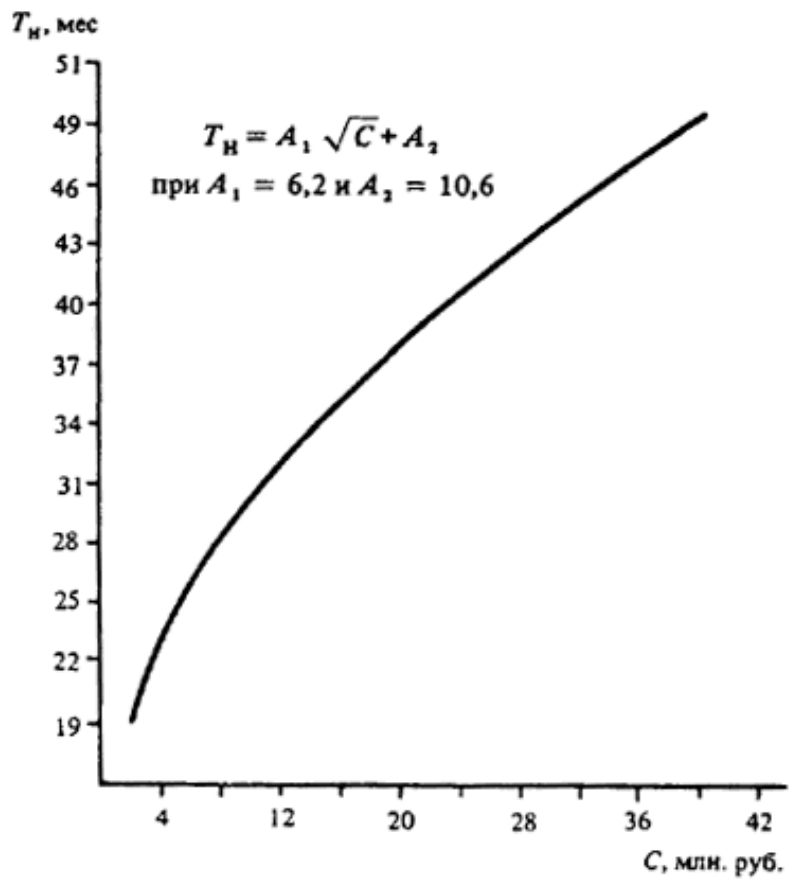
Черт. 21. Определение T_n различных объектов при C = 2 - 40 млн. руб.
