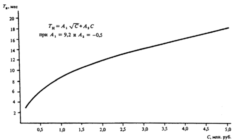
Черт. 5. Определение T_n установок подготовки, газокomppressorных при C = 0,1 - 6,0 млн. руб.
