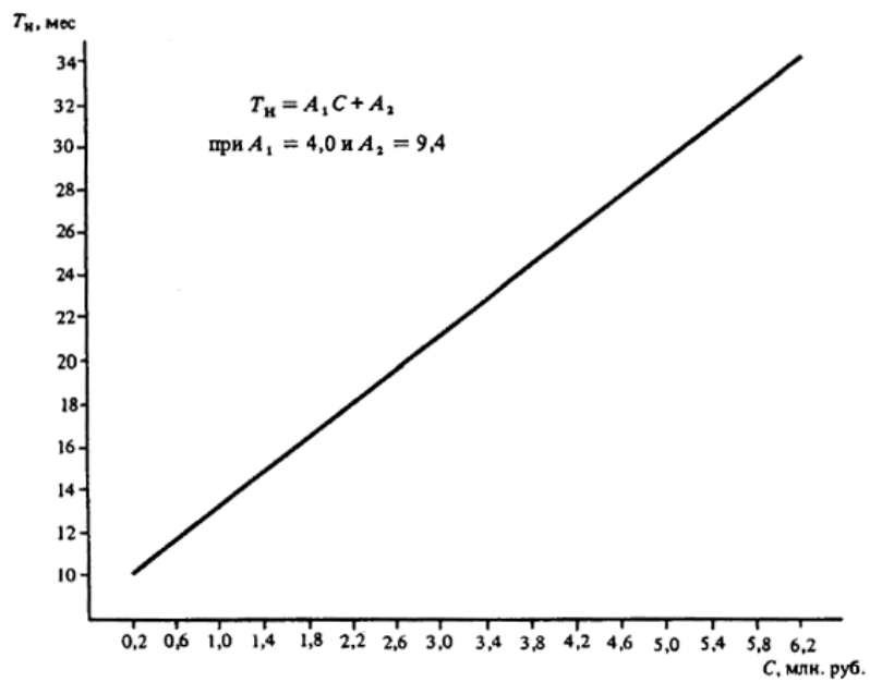
Черт. 53. Определение T_n объектов речного транспорта при C = 0,2 - 6,2 млн. руб.
