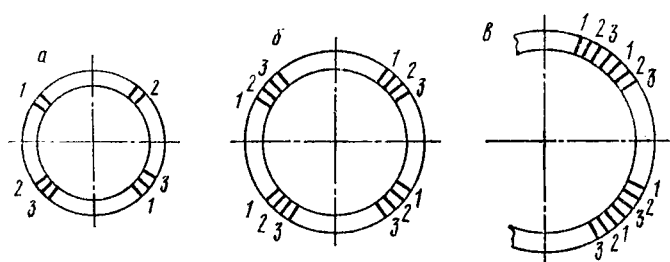
Рис. 3. Схема вырезки образцов для механических испытаний
