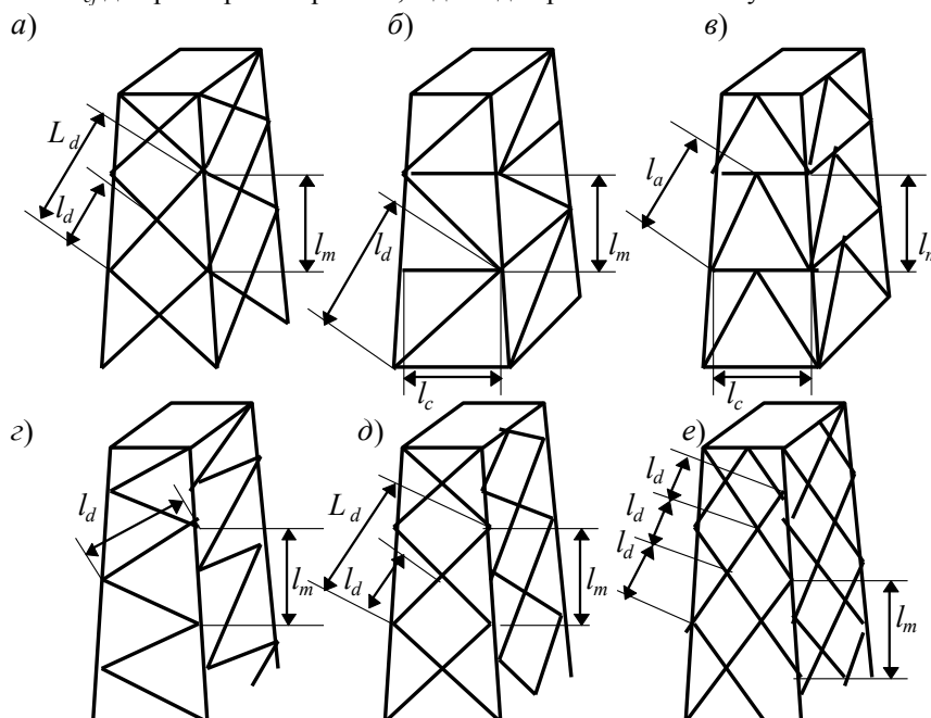
Рис.9*. Схемы пространственных решетчатых конструкций а, б, в – с совмещенными в смежных гранях углами; г, д, е – с несомещенными в смежных гранях углами
