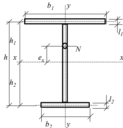
Рис. 27. Схема двутаврового сечения с одной осью симметрии при внешнем сжатии
