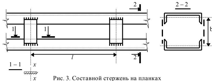
Рис. 3. Составной стержень на планках
