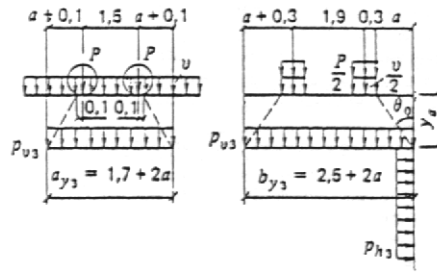
Черт. 4. Схема давления от автомобильной нагрузки АК при движении ее вдоль сооружения
