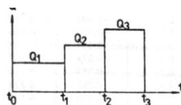
Черт. 2. Ступенчатый график откачки
