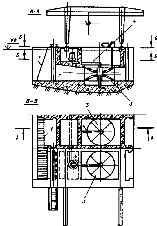
Черт. 9. Конический двухполосный рыбозаградитель с рыбоотводом 1 - сороудерживающая решетка; 2 - камера; 3 - заградитель; 4 - труба рыбоотвода
