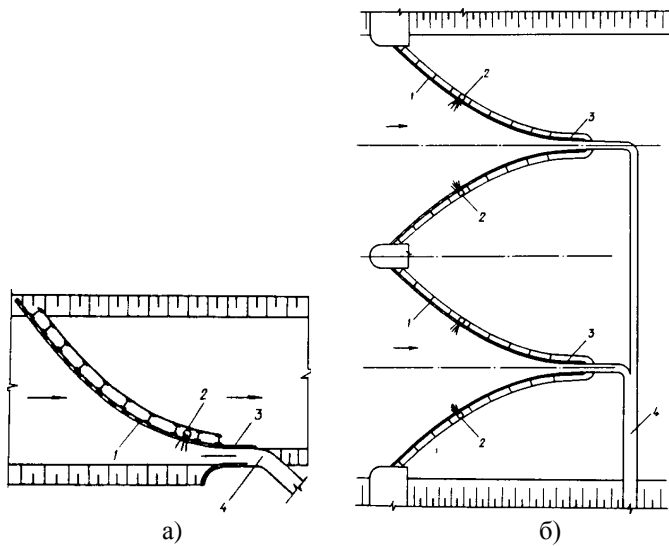
Черт. 11. Вертикальные сетчатые, перфорированные или фильтрующие экраны a - вертикальный экран; б - W - образный экран; 1 - вертикальный экран; 2 - промывное устройство; 3 - глухая часть экране; 4 - рыбоотвод
