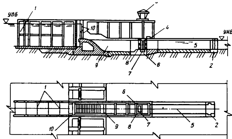
Черт.6. Рыбоподъемные сооружения. Механический рыбоподъемник
