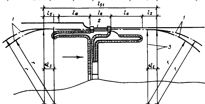
Черт. 1. Схема судоходного шлюза с подходами 1 - ось судового хода; 2 - шлюз; 3 - радиусы поворота судна
