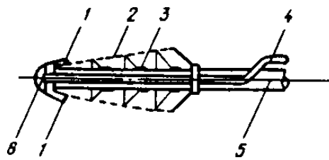
Черт. 8. Оголовок с потокообразователем (РОП)
