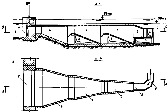
Черт. 13. Рыбозащитный концентратор с вертикальной сепарацией рыб (РКВС) 1 - водозаборный водоем; 2 - оголовок рыбозащитного концентрирующего сооружения; 3 - забральная стенка; 4 - лотки - концентраторы; 5 - оголовок рыбоотвода; 6 - рыбоотвод; 7 - водоприемник; 8 - водозаборные окна; 9 - сопрягающая стенка
