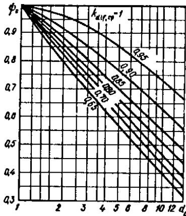
Рис.8. Графики значений коэффициента \psi_c
