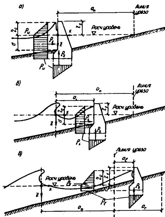
Рис.27. Эпюры волнового давления на вертикальную волнозащитную стену при расположении сооружения: а - в зоне прибойной волны; б - в приурезовой зоне; в - за линией уреза
