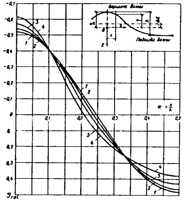
Рис.20. График значений коэффициента \eta_{rel}
