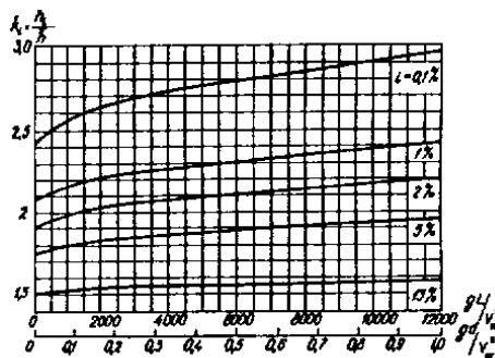
Рис. 2. Графики значений коэффициента k_i
