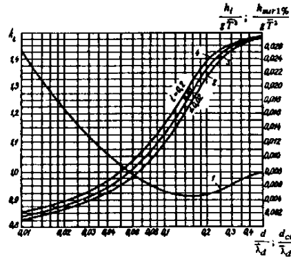
Рис. 5. Графики для определения 1 - коэффициента k_i ; 2,3 и 4- величины d_{cr} / \bar{\lambda}_d
