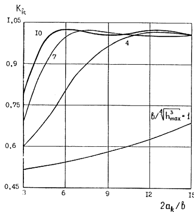
Рис.44. Графики значений коэффициента K_k
