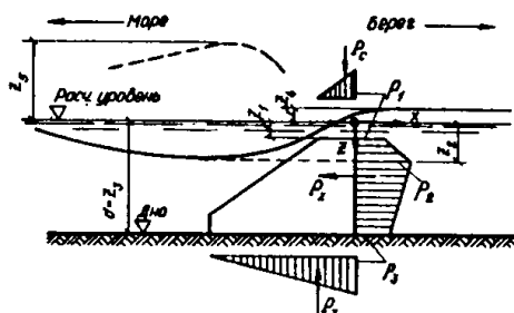
Рис.26. Эпюры волнового давления на подводный волнолом
