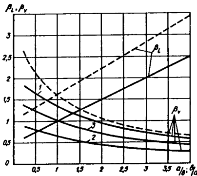
Рис 17. Графики значений инерционного \beta_i и скоростного коэффициентов формы (для эллиптических преград - сплошные линии, при призматических - штриховые линии) в зависимости от \alpha/b (для Q , q и P_x ) или b/\alpha (для P_z ) 1 - для шероховатой эллиптической преграды; 2 - гладкой; 3 - шероховатой в подводной и гладкой в надводной частях вертикальной эллиптической преграды
