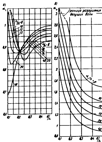
Рис 16. Графики значений инерционного \alpha_i и скоростного \alpha_v коэффициентов глубины
