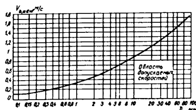
Рис.7. График допустимых значений неразрывающихся донных скоростей
