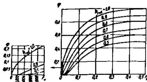
Рис. 36. Графики значений коэффициента \varphi
