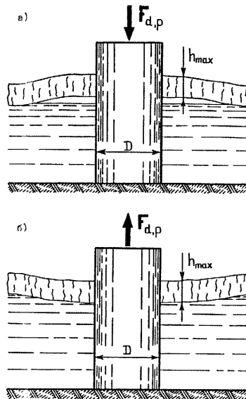
Рис.42. Схемы приложения нагрузки от примерзшего к отдельно стоящей опоре ледяного покрова при изменении уровня воды (УВ) а - при понижении УВ; б - при повышении УВ
