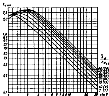
Рис. 10*. Графики значений коэффициента k_{гун}
