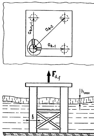
Рис.43. Схемы приложения нагрузки от примерзшего к сооружению из системы вертикальных колонн ледяного покрова при повышении уровня воды Примечание. При понижении уровня воды сила F_{d,ψ} направлена вниз
