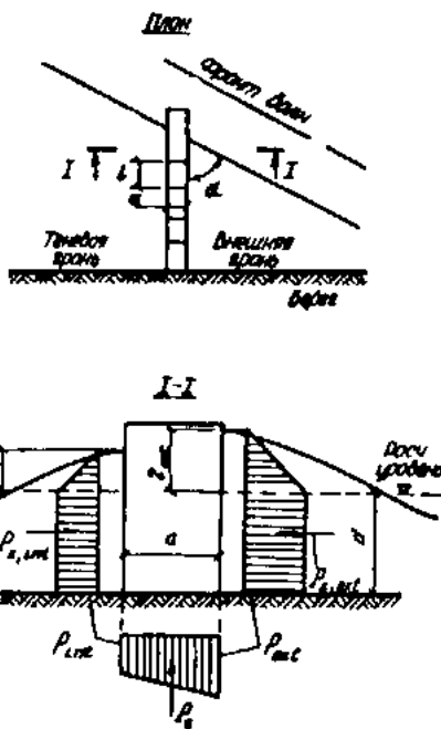
Рис. 30. Эпюры волнового давления на буну
