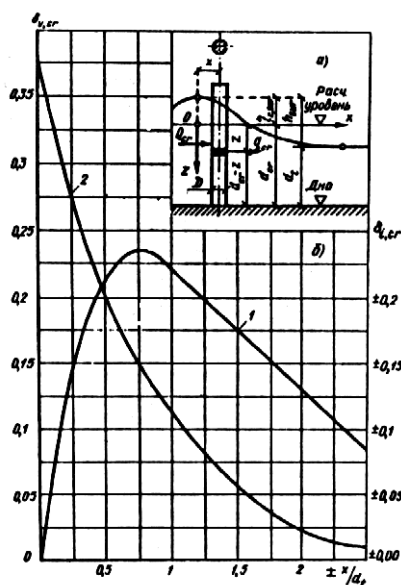
Рис. 24. Схема к определению нагрузок от разбивающихся волн и графики значений коэффициентов \delta_{i,cr} - кривая 1 и \delta_{v,cr} - кривая 2
