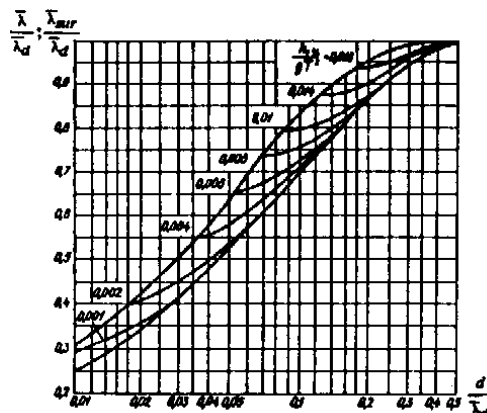
Рис. 4. Графики для определения значений \lambda/\lambda_d в мелководной и \lambda_{sur}/\lambda_d в прибойной зонах
