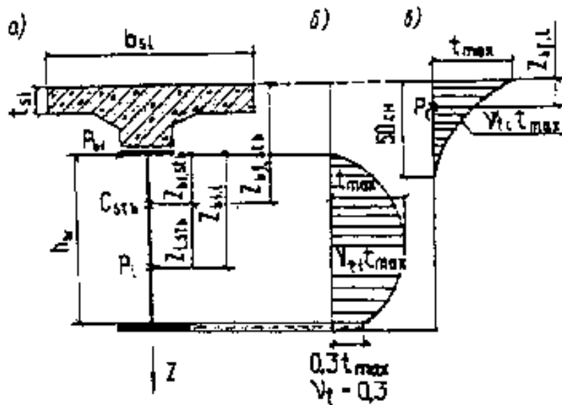
Черт. 14. Поперечное сечение сталежелезобетонной конструкции и расчетные эпюры разности температур
