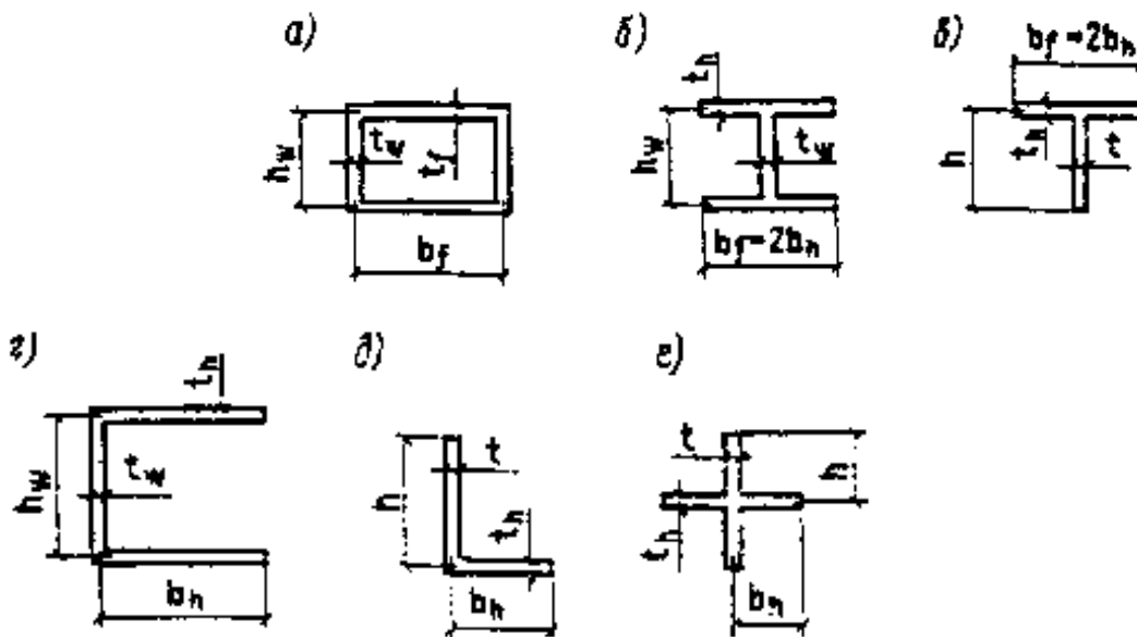
Черт. 11. Схемы расчетных сечений элементов, не подкрепленных ребрами жесткости
