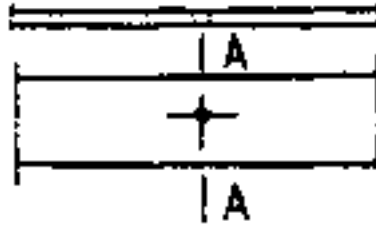
Черт. 1. Расположение проверяемого на выносливость расчетного сечения А—А по основному металлу в сечениях нетто по соединительным болтам составных элементов, а также у свободного отверстия
