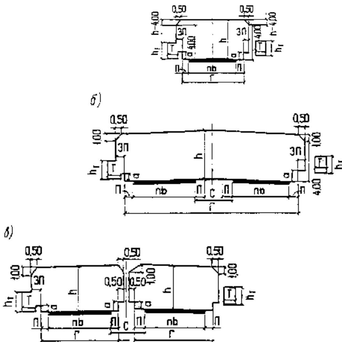
Черт. 1. Схемы габаритов приближения конструкций на автодорожных и городских мостах
