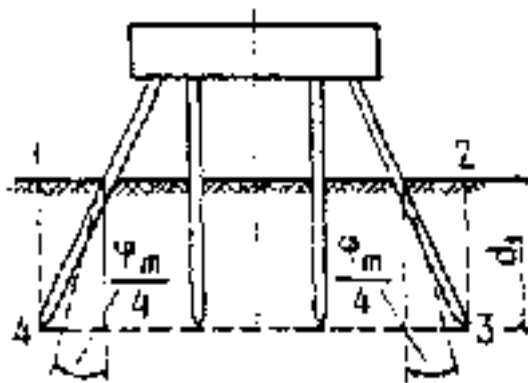
Черт. 3. Условный свайный фундамент с ростверком, расположенным над грунтом при угле наклона свай менее \varphi_m/4
