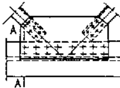
Черт. 3. Расположение проверяемого на выносливость расчетного сечения А—А по основному металлу в сечении брутто по первому ряду высокопрочных болтов в прикреплении фасонки к несъёмным в данном узле поясам сплошных балок и элементам решетчатых форм
