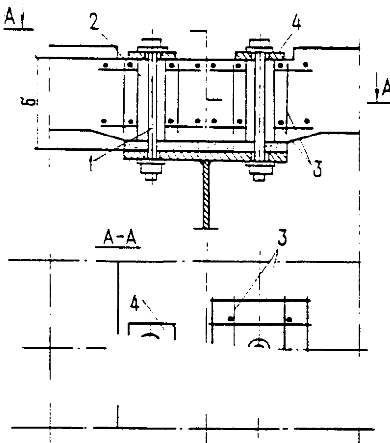
Конструкция болтового объединения
