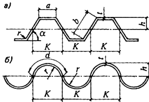
Черт. 12. Расчетная схема сжатого гофрированного листа
