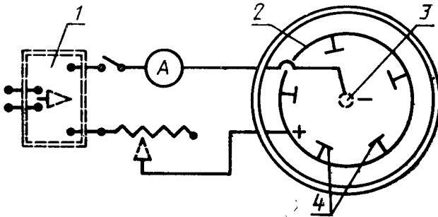
Схема установки катодной очистки пластин
