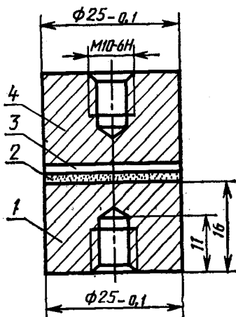
1 — образец; 2 — покрытие; 3 — клеевая прослойка; 4 — контрообразец
