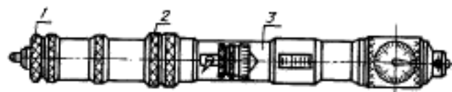
1 — измерительный наконечник; 2 — удлинитель; 3 — микрометрическая головка с индикатором
