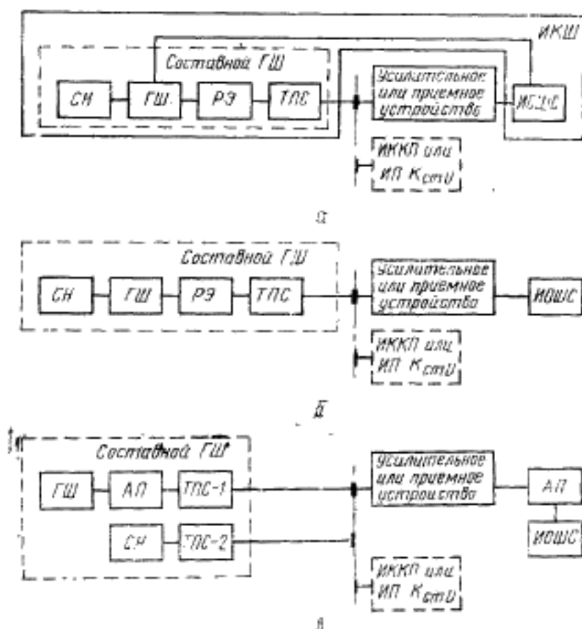
а - схема стенда для измерения коэффициента шума с использованием промодулированного генератора шума (ГШ); б - то же, источником двух отсчетов; в - схема стенда для прецизионных измерений с использованием аттестованного поляризационного аттенюатора (АП)
