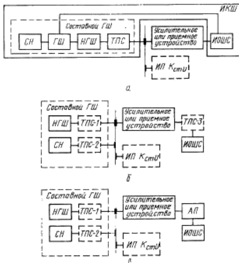
а—схема стенда для измерения ЭИТВ устройств с использованием НГШ проходного типа и ИКШ в автоматическом режиме; б—то же, с использованием НГШ непроходного типа; в—схема стенда для прецизионных измерений
