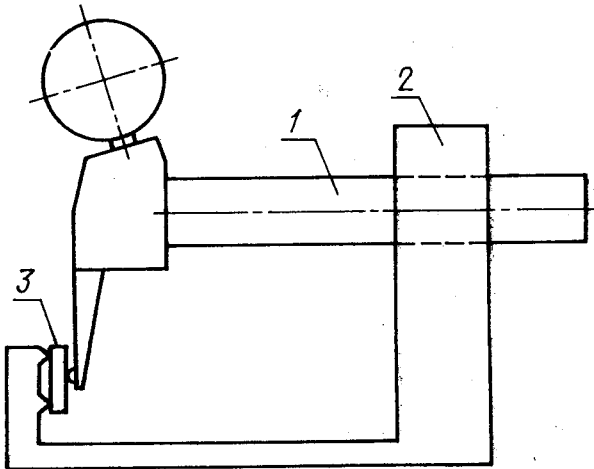
1—шагомер; 2—стойка С-II по ГОСТ 10197—70; 3—плоско-параллельная концевая мера длины
