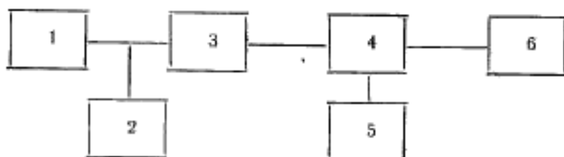
1—генератор СВЧ; 2—частотомер; 3—развязывающий аттенюатор и ферритовый вентиль; 4—измерительная линия; 5—индикатор измерительной линии; 6—поверяемый ваттметр
