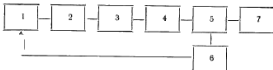
1—генератор СВЧ; 2—развязывающий аттенюатор или ферритовый вентиль; 3—регулируемый аттенюатор; 4—поверяемый ваттметр; 5—измерительная линия; 6—компаратор импульсной мощности; 7—волновый короткозамыкатель
