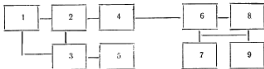
1—генератор СВЧ; 2—детекторный преобразователь компаратора импульсной мощности; 3—компаратор импульсной мощности; 4—диод; 5—осциллограф; 6—калибратор мощности; 7—термисторный мост; 8—поверяемый ваттметр; 9—вольтметр
