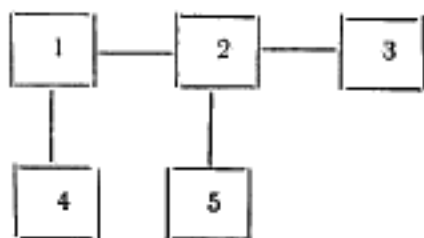
1 — развязывающее устройство; 2 — поверяемая измерительная линия; 3 — короткозамкнутая нагрузка; 4 — генератор сигналов; 5 — индикаторный прибор поверяемой линии
