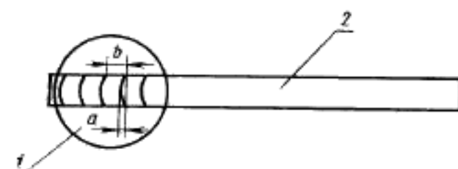
1—плоская стеклянная пластина; 2—контрольный брусок
