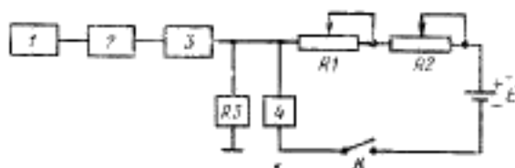
1—поверяемый генератор; 2—измерительный attenuator; 3—детекторная головка; 4—фотокомпенсационный микровольтметр типа Ф 116/2; R_1 , R_2 —переменные резисторы типа СП1; R_3 —резистор 3 кОм, 0,5 Вт; K —ключ; E —источник постоянного тока.
