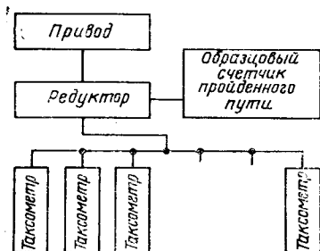
Структурная схема установки для поверки таксометров.
