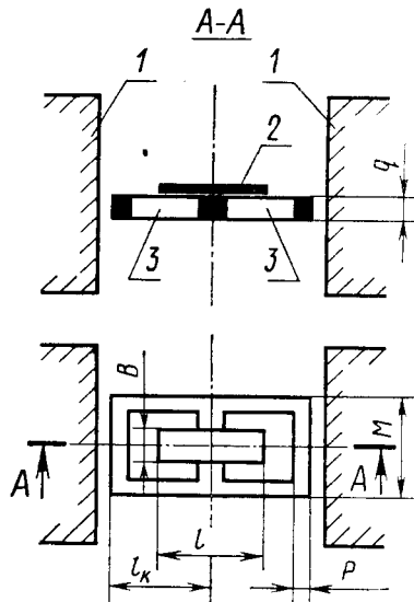
1—полюсные наконечники электромагнита; 2—образец; 3—катушки индукционного преобразователя
