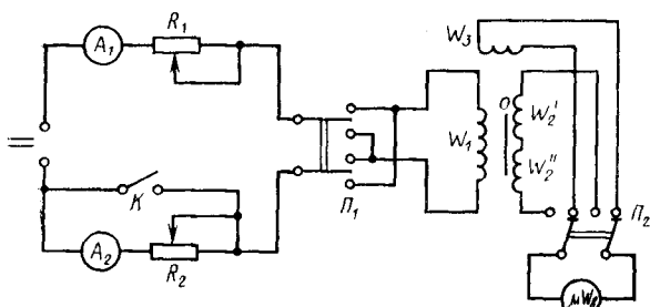
R_1, R_2 — регулировочные реостаты; A_1, A_2 — амперметры; K — ключ; P_1, P_2 — двухполюсные переключатели; W_2: W_2' — катушки индукционного преобразователя для измерения магнитного потока; W_3 — измерительная катушка; W_1 — обмотка намагничивающего устройства; \mu W — микроамперметр; O — образец.
