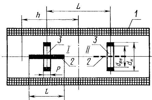
1—соленоид; 2—образец; 3—катушки индукционного преобразователя.
