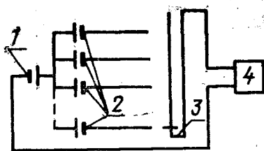
1—образцовый Н. Э.; 2—поверяемый Н. Э.; 3—коммутатор Н. Э.; 4—прибор для определения э.д.с. (потенциометр, цифровой вольтметр)
