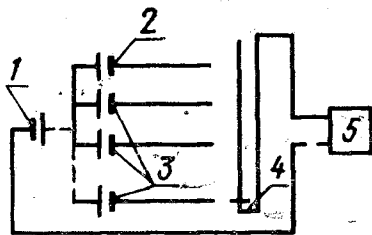
1—вспомогательный Н. Э.; 2—образцовый Н. Э.; 3—поверяемые Н. Э.; 4—коммутатор Н. Э.; 5—прибор для определения э.д.с.
