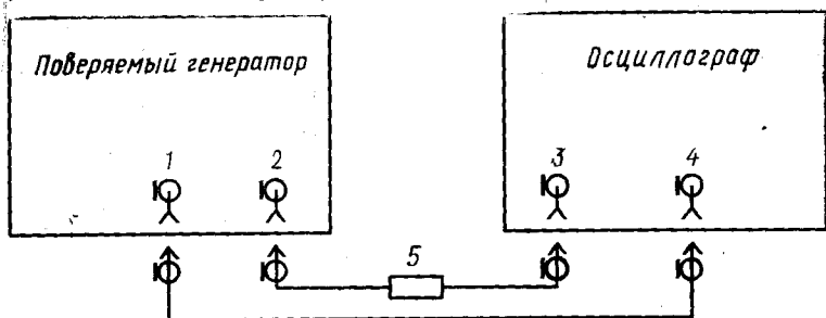
1—выход основных импульсов канала I; 2—выход основных импульсов канала II; 3—вход канала Y; 4—вход синхронизирующих импульсов; 5—аттенюатор Черт. 3
