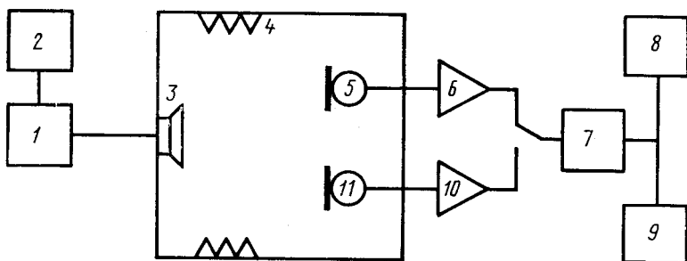
1—генератор; 2—частотомер; 3—громкоговоритель; 4—заглушенная камера; 5 и 11—образцовый и проверяемый микрофоны; 6 и 10—микрофонные усилители; 7—магазин затухания; 8—электронный вольтметр; 9—осциллограф.
