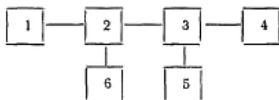
1—измерительный генератор; 2, 3—коаксиальный соединитель; 4—поверяемый вольтметр; 5—образцовый вольтметр; 6—образцовый частотомер
