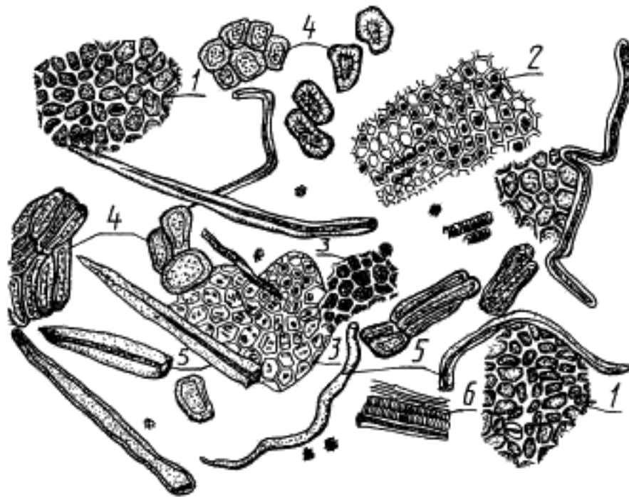
Строение плода шиповника (увеличение 280 x )
