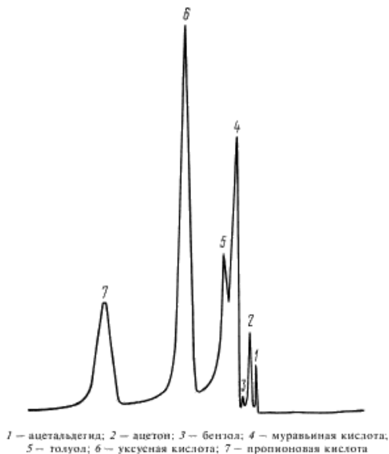
Типовая хроматограмма технической муравьиной кислоты
