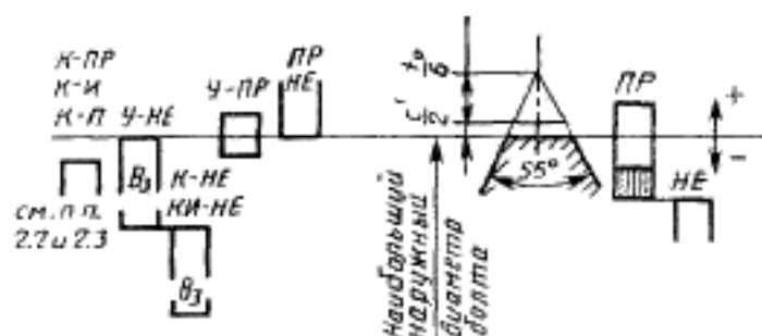
Калибры для контроля болтов (наружной резьбы)
