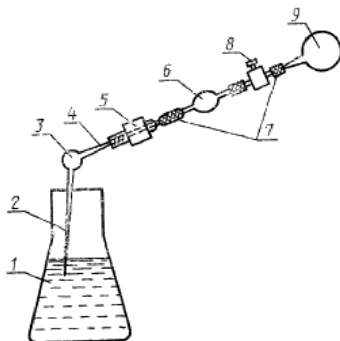
1—колба с меляжем; 2, 3—капиллярные концы ампулы; 3—ампула; 5—фторопластовый мундштук; 6—спеклянный индикатор; 7—гибкий шланг; 8—вентиль; 9—резиновая груша
