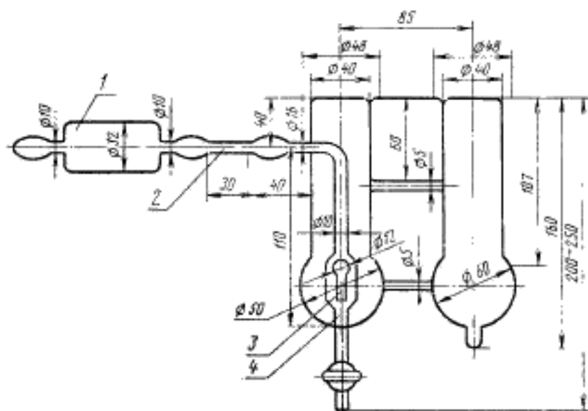
1—вылеулловитель; 2—резиновая трубка; 3—воплавок; 4—четыре отверстия \varnothing 1,5 мм
