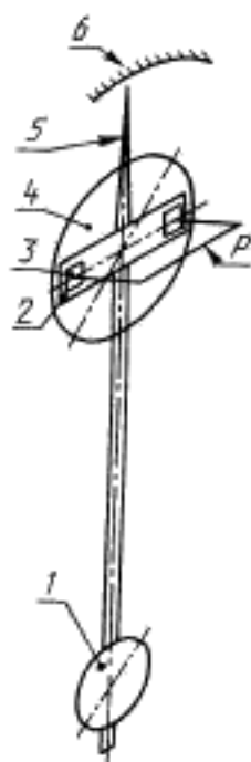
1 — маховик; 2 — держатель образцов; 3 — образцы; 4 — металлическое контртело; 5 — стрелка; 6 — шкала момента трения
