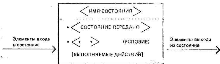
Пример нотации диаграммы переходов состояний
