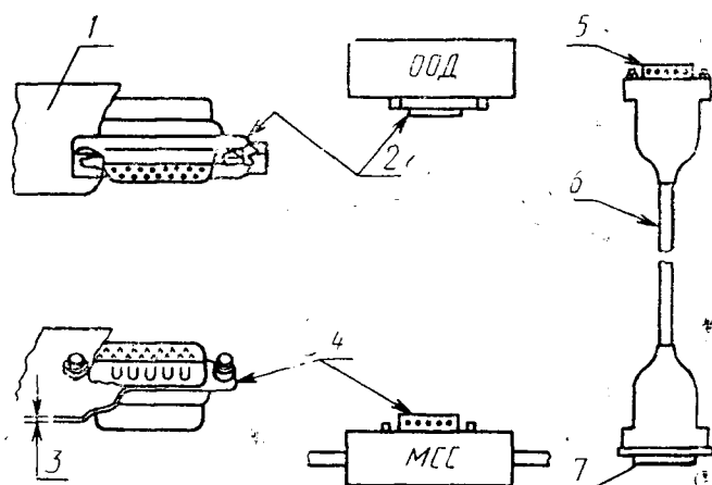
Детали соединителя и конфигурации кабеля ИМС
