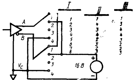
Неисправные состояния генератора
