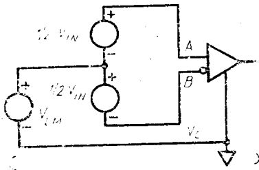
V_{IN} — входное напряжение; V_{CM} — общее напряжение Черт. 7.15
