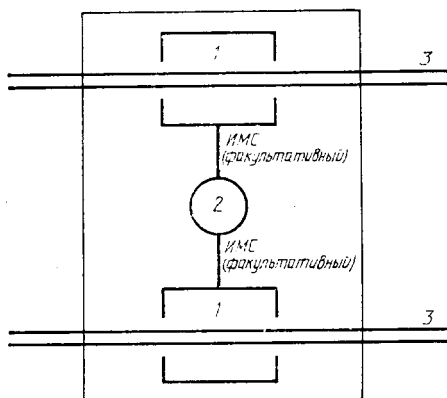
Повторительная установка, конфигурация коаксиал — коаксиал
