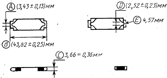
Скользящая защелка соединителя (максимальный размер материала 24)
