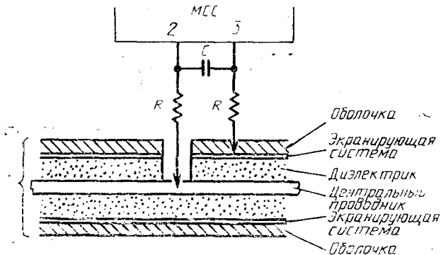
Типовая схема коаксиального ответвительного соединения
