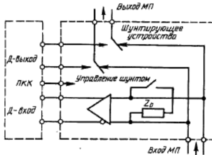
Пример переключения шунта для одного сигнала D-порта
