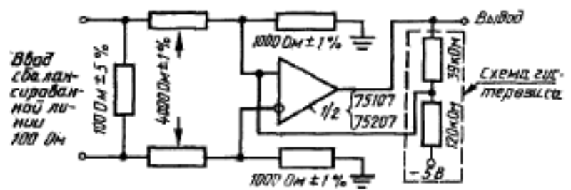
Пример приемника с гистерезисом, дополненным внешними резисторами
