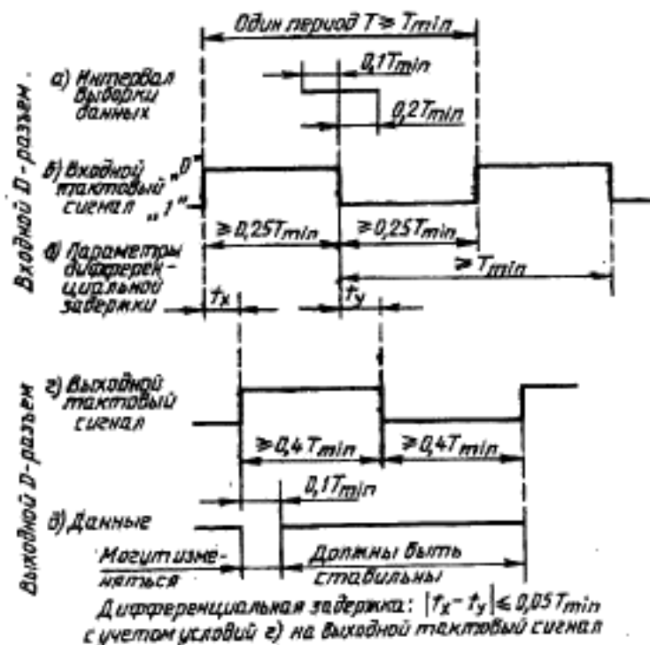
Временные соотношения для сигналов данных и тактовых (информационных и синхронизирующих) на D-соединителях
