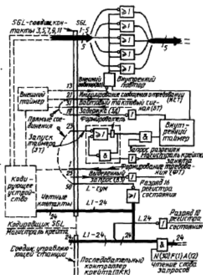
Пример схемы взаимодействия ПКК и кодировщика
