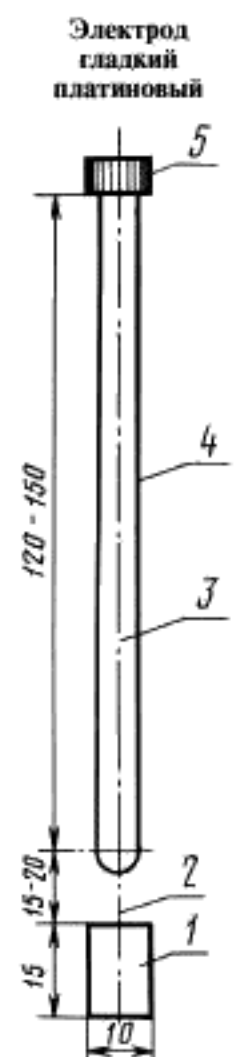
1 — пластинка платиновая; 2 — проволока платиновая; 3 — проволока медная; 4 — трубка стеклянная; 5 — клемма медная
