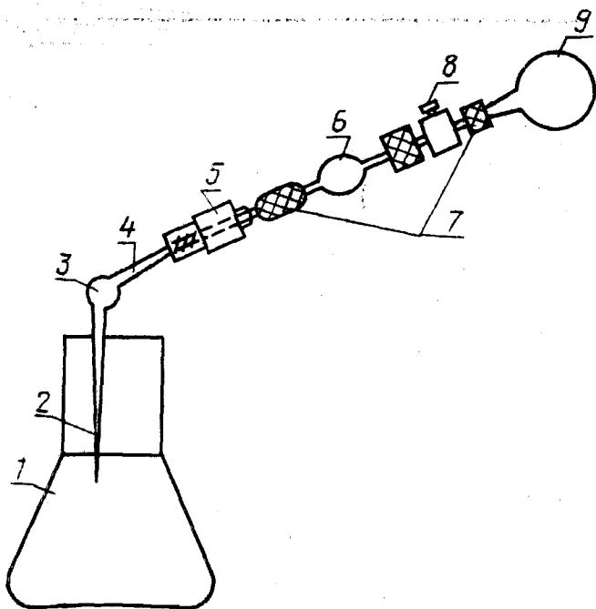
1—колба с кислотой; 2, 4—капиллярные концы ампулы; 3—ампула; 5—фторопластовый мундштук; 6—стеклянный индикатор; 7—гибкий шланг; 8—вентиль; 9—резиновая груша
