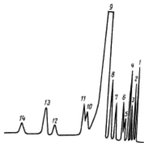
Типовая хроматограмма образца хлорбензола
