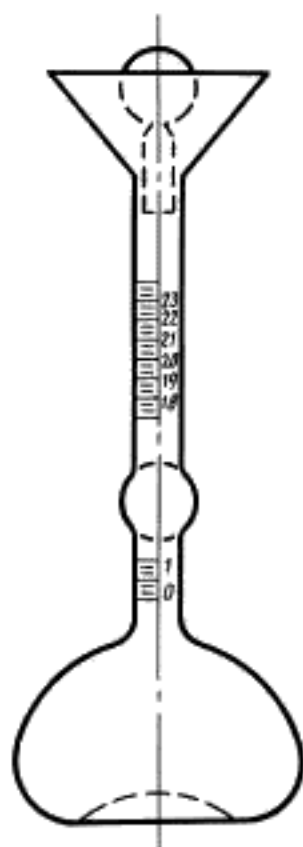
Прибор для определения плотности цемента
