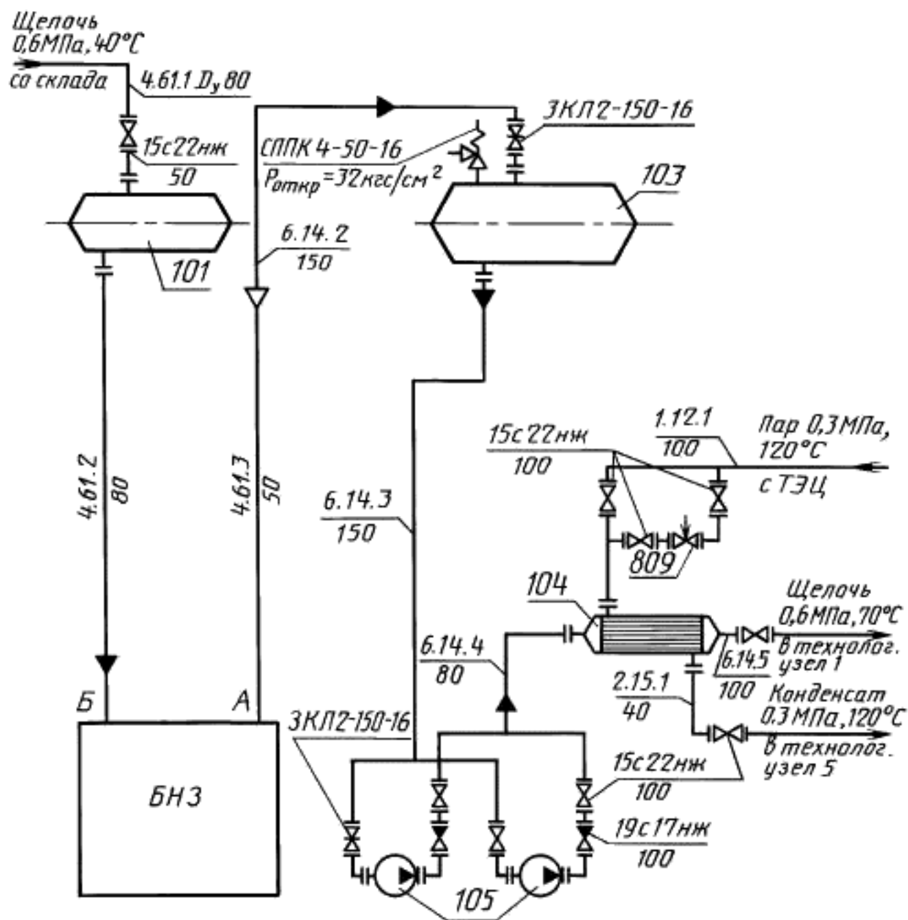
Схема соединений (монтажная)
