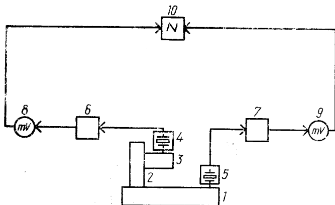
1 — стол вибростенда; 2 — приспособление для испытания; 3 — испытываемое изделие; 4, 5 — пьезоэлектрические вибропреобразователи; 6, 7 — катодные повторители; 8, 9 — милливольтметры; 10 — осциллограф
