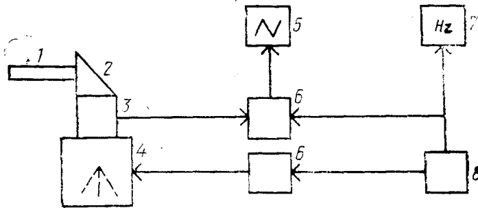
1 — испытываемое изделие; 2 — согласующий держатель; 3 — пьезоэлектрический детектор резонансных частот; 4 — вибратор; 5 — индикатор (осциллограф); 6 — усилитель; 7 — частотомер; 8 — генератор звуковых частот
