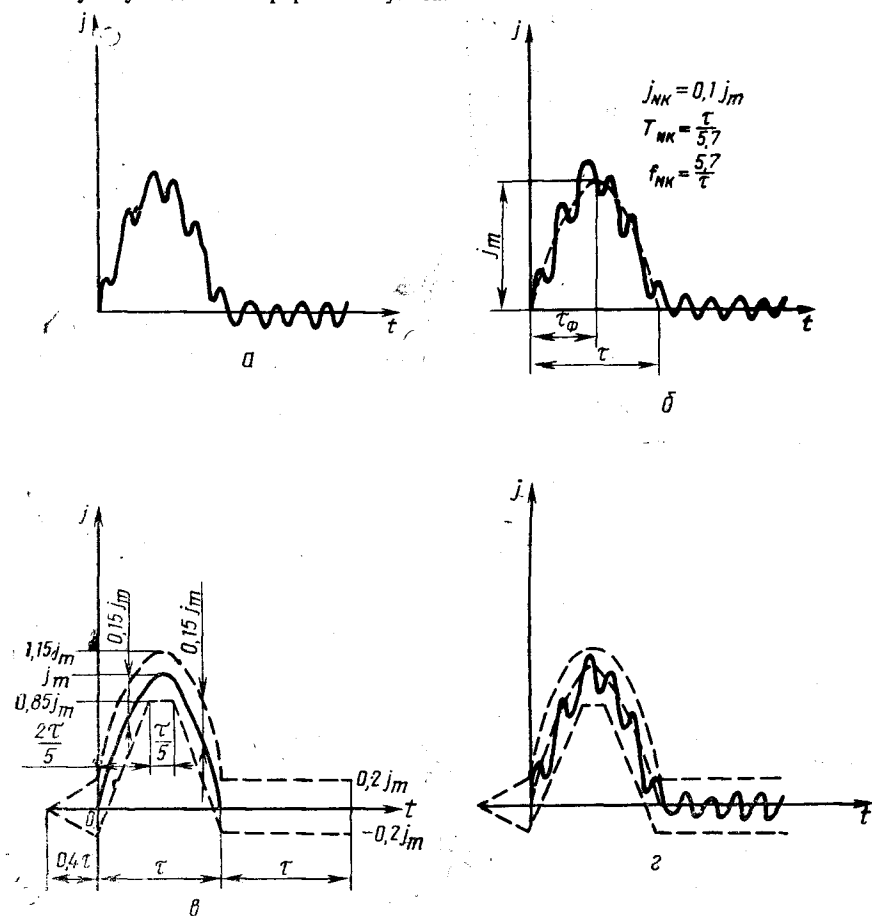
а — осциллограмма исходного импульса, б — выявление усредненного профиля импульса; в — нормированная форма импульса; г — оценка формы импульса
