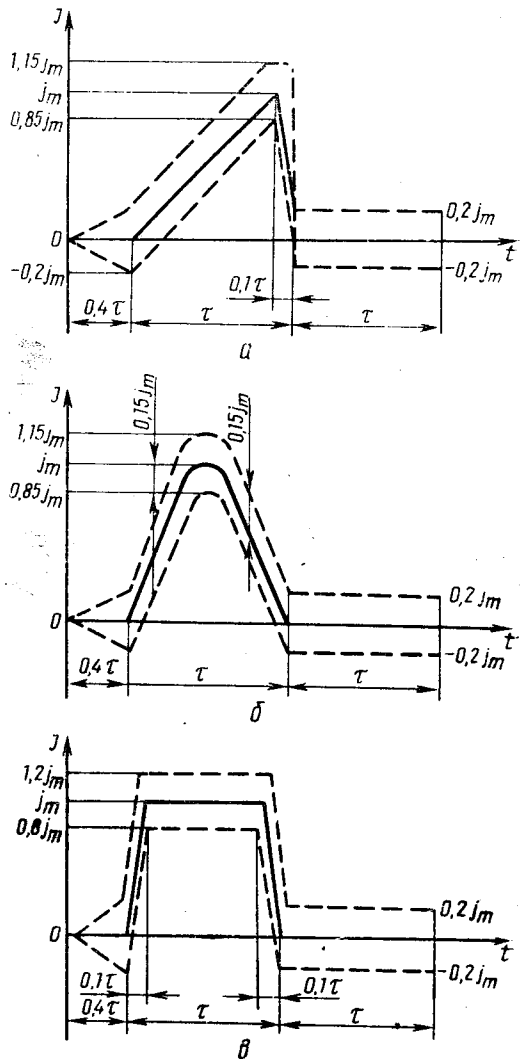
а — псевдоимпульс; б — полусинусоидальный импульс; в — трапецидальный импульс; --- границы допусков
