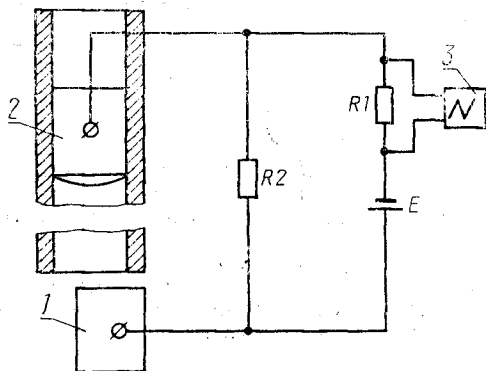
1 — наковальня (основание); 2 — блок (стол); 3 — осциллограф
