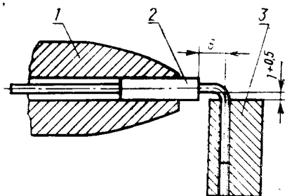
Испытание гибких проволочных выводов на скручивание
