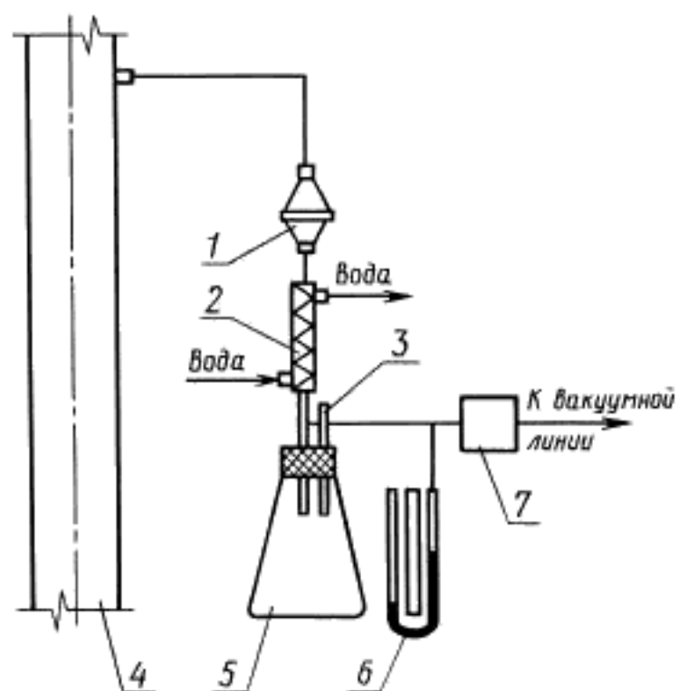
СХЕМА установки приборов для определения влажности газа конденсационным методом
