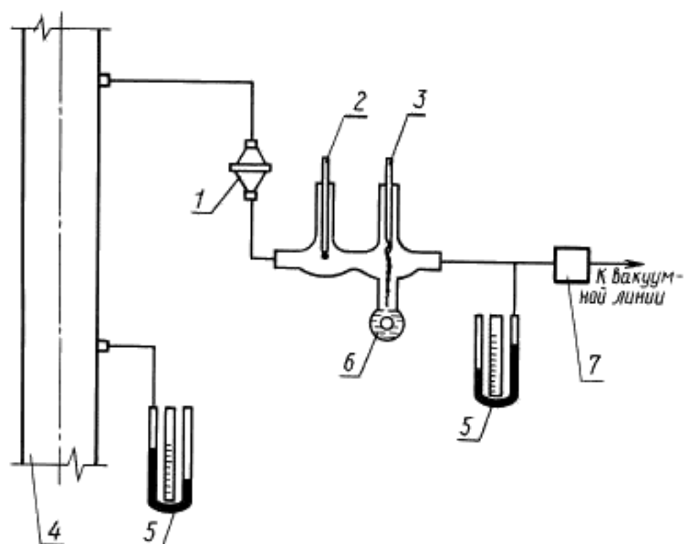
СХЕМА установки приборов для определения влажности газа психрометрическим методом
