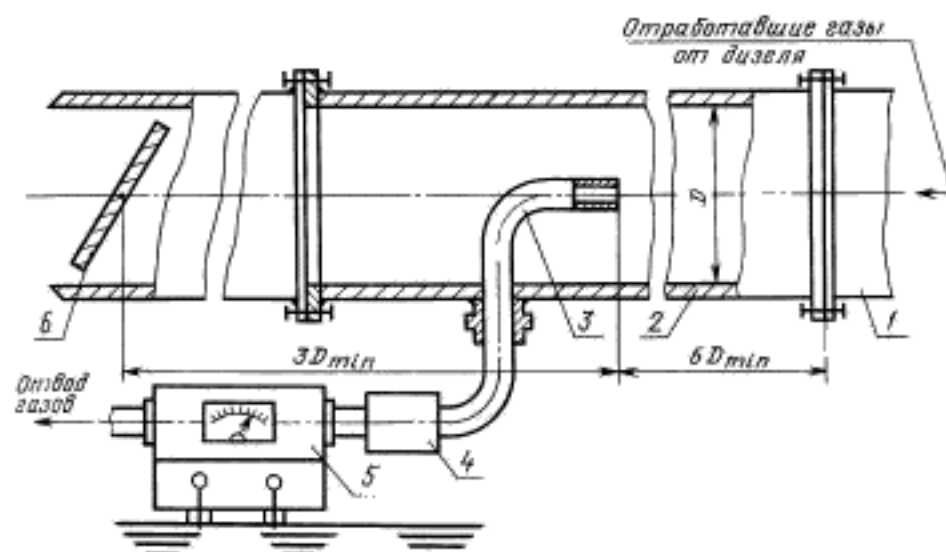
1 — выхлопной трубопровод дизеля; 2 — выхлопная труба испытательного стенда; 3 — газоотборник дымомера; 4 — ресивер; 5 — измерительный прибор; 6 — регулирующая заслонка
