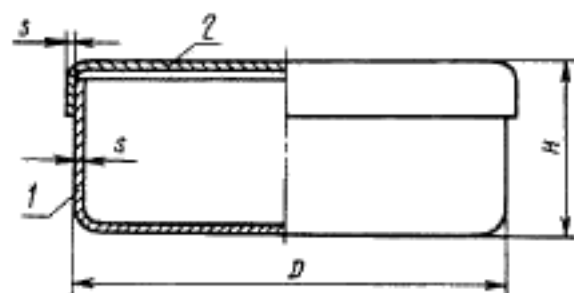
1 — корпус; 2 — крышка
