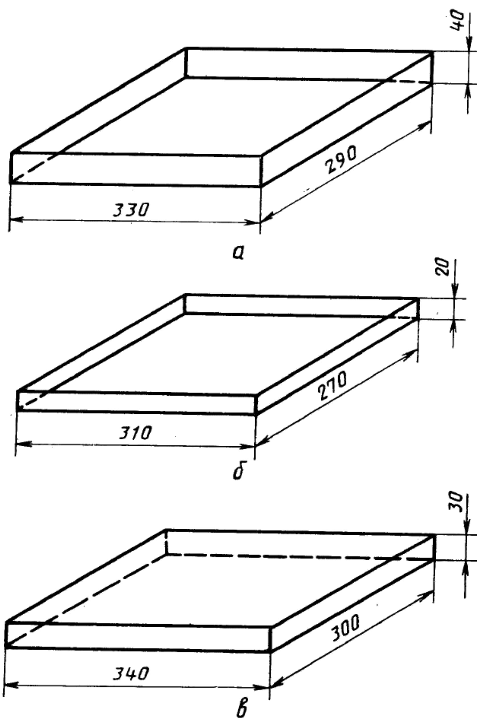
a —поддон; б —прижимная рамка; в —крышка
