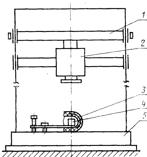
1—каретка; 2—боек; 3—носок; 4—пластилиновый столбик; 5—основание
