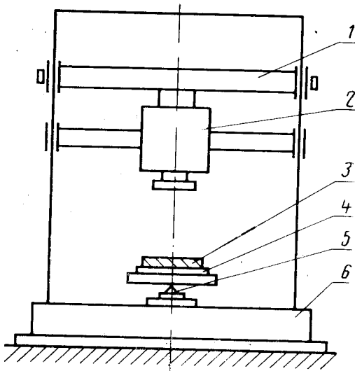
1—каретка; 2—боек; 3—защитный элемент; 4—плита; 5—датчик; 6—основание
