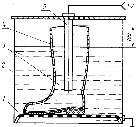
1—сетка; 2—ванна; 3—электролит; 4—образец; 5—электрод
