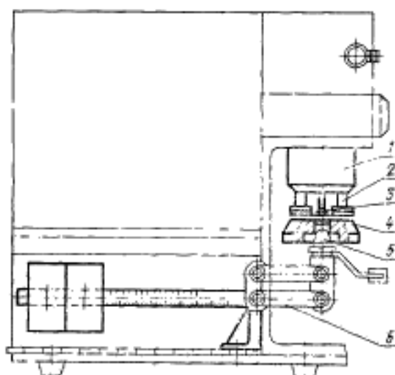
1 — истирающая головка; 2 — бегунок; 3 — устройство для натяжения испытуемой или абразивной ткани; 4 — вялец; 5 — опора вялец; 6 — рычажно-грузовая система для создания нормального давления
