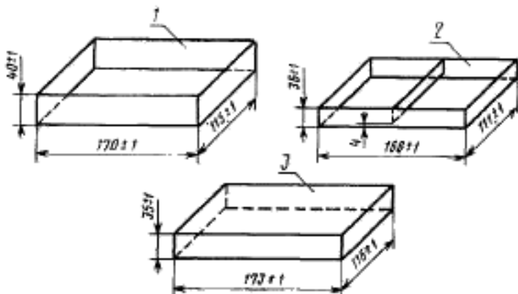
1—металлическая кювета; 2—прижимная рамка; 3—крышка
